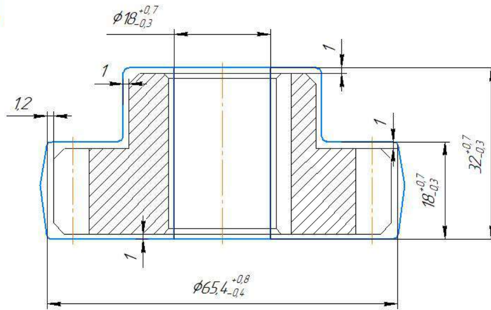
Схема розміщення полів припусків
