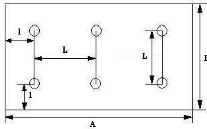
Рисунок 8.1 – Схема розміщення світильників
