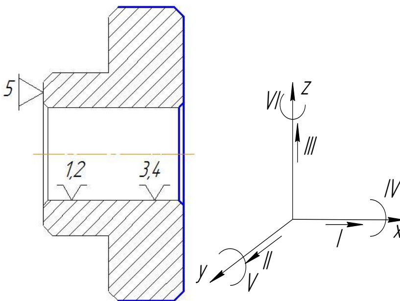
Рисунок 6.2 – Схема базування заготовки на токарно-багаторіздцевій операції
