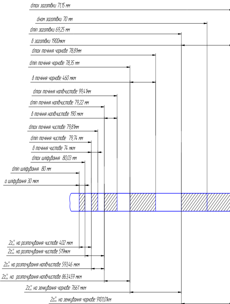
Рисунок 6.1 – Схема графічного розташування припусків і допусків на обробку зовнішньої поверхні
