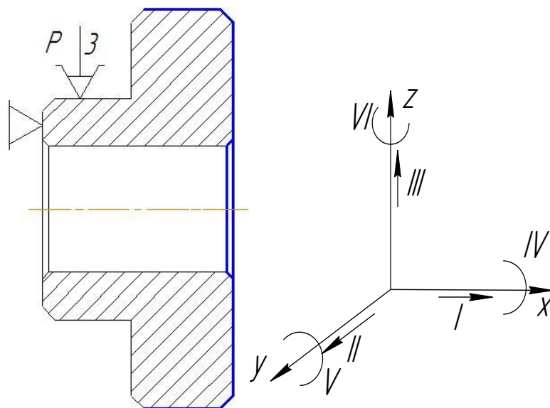
Рисунок 6.2 – Схема базування заготовки на токарно-багаторіздевій операції
