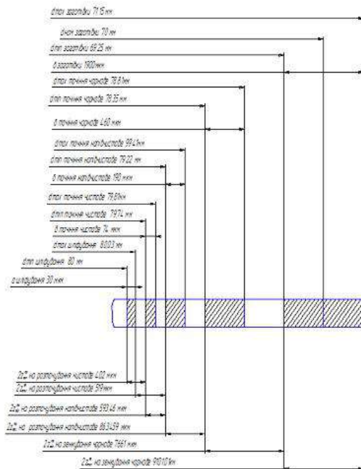
Схема розміщення полів припусків
