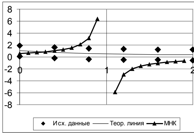
Рисунок 2 – Теоретическая регрессия y = 1/(1 + x) и эмпирическая функция регрессии \hat{y} = 1/(1,63218-1,63863x) , найденная по МНК после линеаризации
