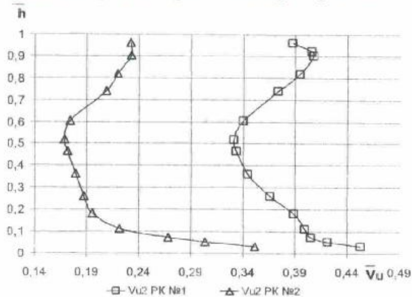
Рис. 6. Графіки колової складової абсолютної швидкості на оптимальному режимі на виході з РК №1 та РК №2.
