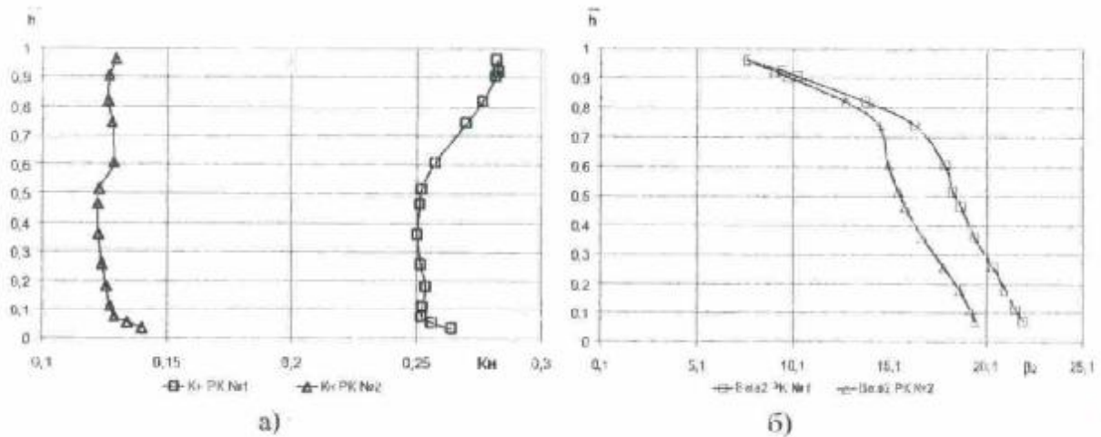
Рис. 7. а) Графік розподілу коефіцієнта напору вздовж висоти лопасті на оптимальному режимі для РК №1 та РК №2; б) Графік розподілу кута потоку на оптимальному режимі на виході з РК №1 та РК №2
