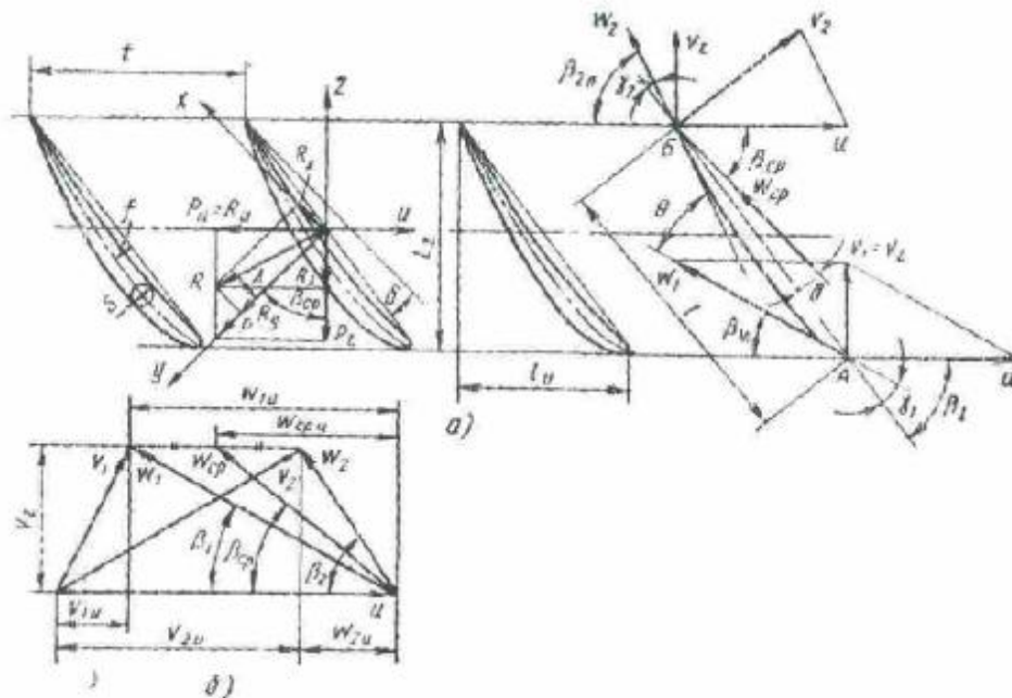
Рис. 2. Параметри ґратки профілів осьового колеса [9]
