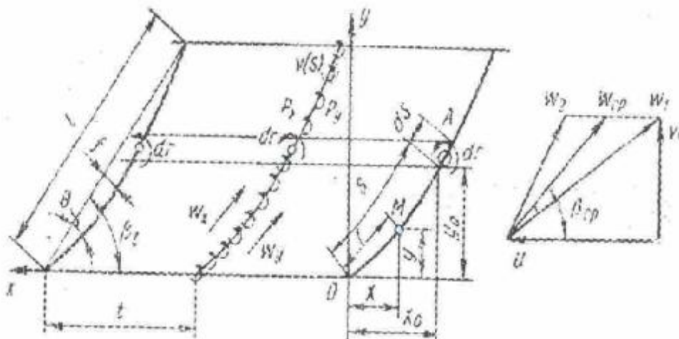
Рис. 1. Схема для розрахунку ґратки профілів методом І.М. Вознесенського – В.Ф. Пекіна [9]
