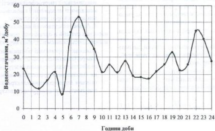
Рис. 2. Графік водопостачання на ЦТП-17 м. Суми за 13.02.2008 року.
