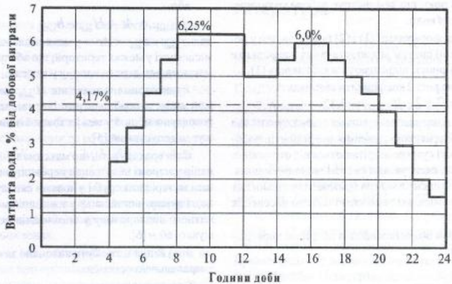
Рис. 1. Ступеневий графік добового водоспоживання для середнього міста.
