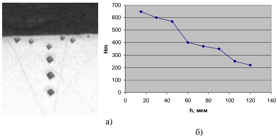
Рисунок 12 - Микрошлиф (а) и распределение микротвердости в поверхностном слое стали 40X образца №3 (б)
