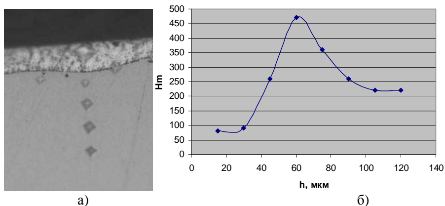
Рисунок 13 - Микрошлиф (а) и распределение микротвердости в поверхностном слое стали 40X образца № 4 (б)
