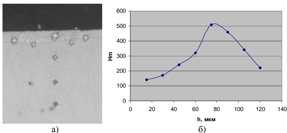
Рисунок 14 - Микрошлиф (а) и распределение микротвердости в поверхностном слое стали 40X образца №5 (б)
