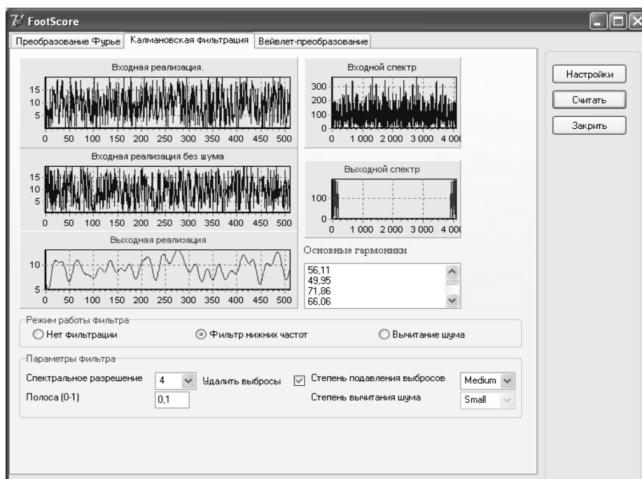
Рис. 7. Видяк вкладки «Калмановская фильтрация»
