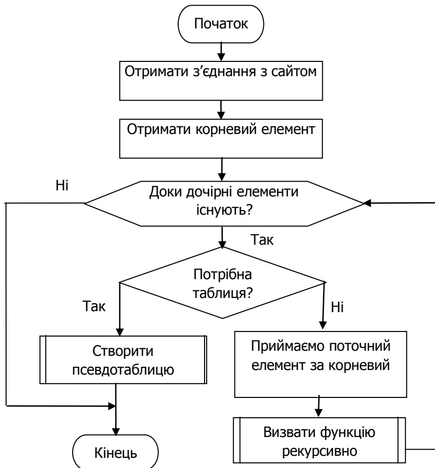
Рис. 1. Алгоритм зчитування даних
