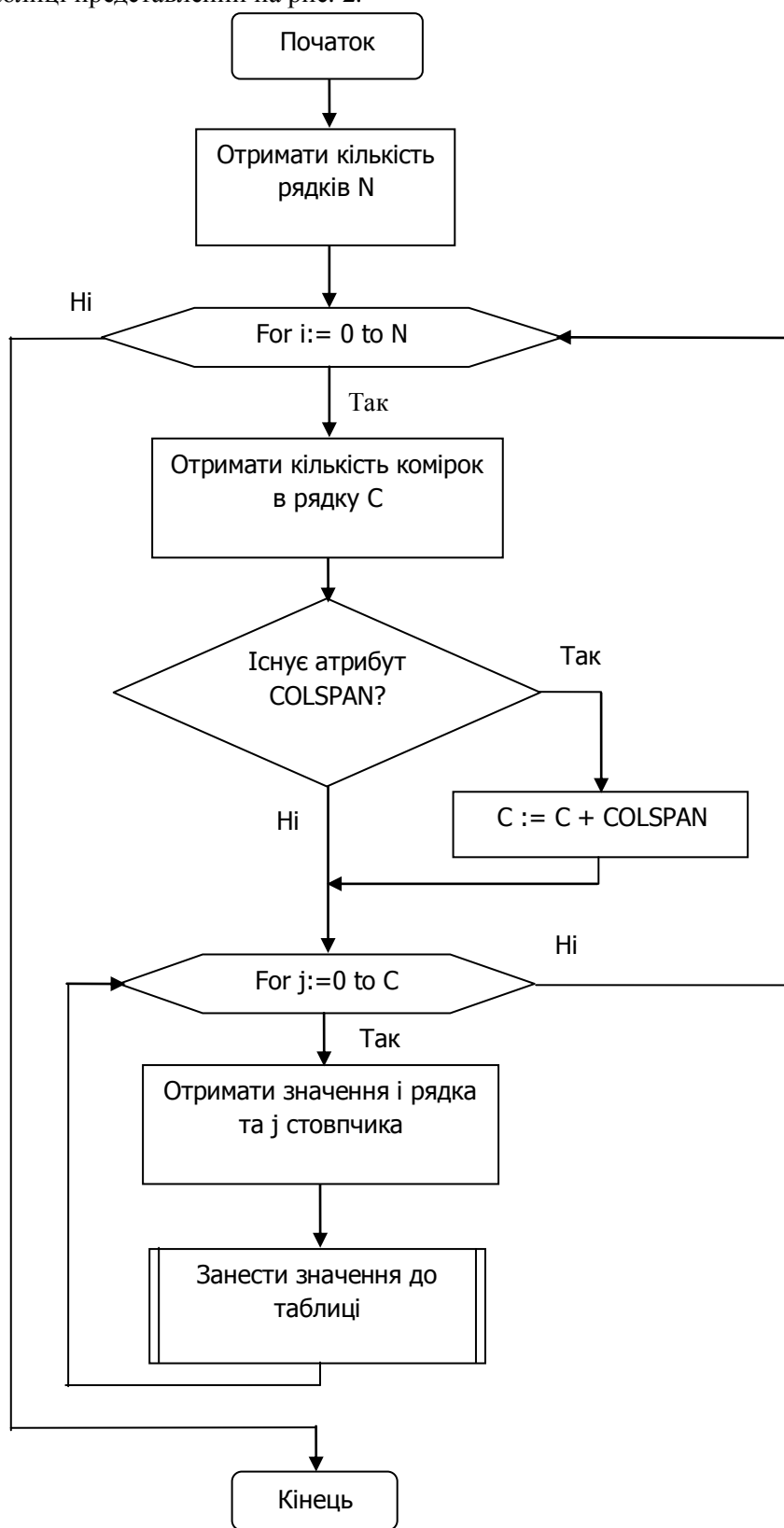
Рис. 2. Алгоритм роботи парсера при створенні псевдотаблиці
