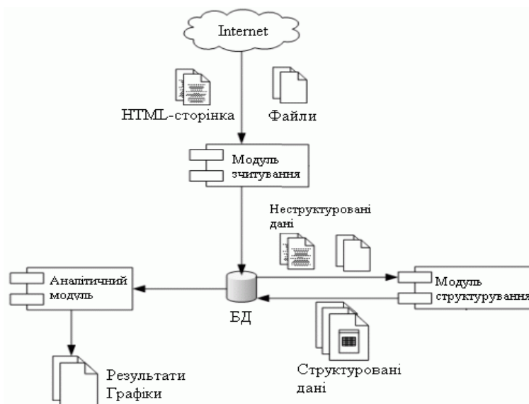
Рис. 3. Схема роботи системи збирання, розміщення та аналізу даних
