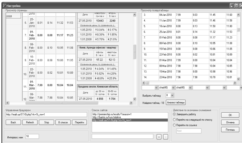
Рис. 5. Діалогове вікно «Настройка»
