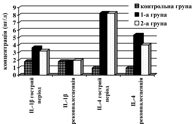
Мал. 5. Рівні вмісту ІЛ-1 \beta і ІЛ 4 у пацієнтів досліджуваних груп
