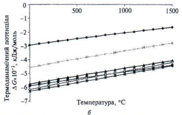
Рис. 2. Залежність термодинамічного потенціалу від температури при окисненні карбіду титану (а): \bullet – реакція (1); \blacksquare – реакція (2); \blacktriangle – реакція (3); \blacklozenge – реакція (4); \blacktriangledown – реакція (5); і хрому (б): \bullet – реакція (6); \blacksquare – реакція (7); \blacktriangle – реакція (8); \blacklozenge – реакція (9); \blacktriangledown – реакція (10); \star – реакція (11); \circ – реакція (12)
