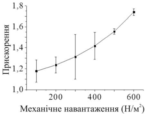
Рис. 4. Залежність прискорення дифузії від навантаження
