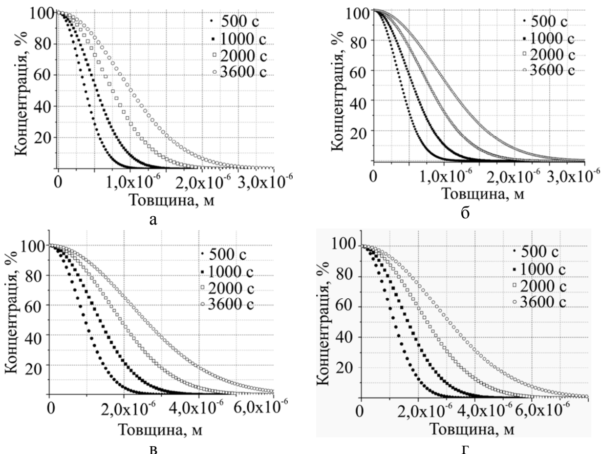
Рис.10. Залежність концентрації дифузанта від глибини дифузійного шару при дифузії Ni в Cu: а) при температурі 1000 К; б) при температурі 1200 К; Au в Cu: в) при температурі 1000 К; г) при температурі 1200 К
