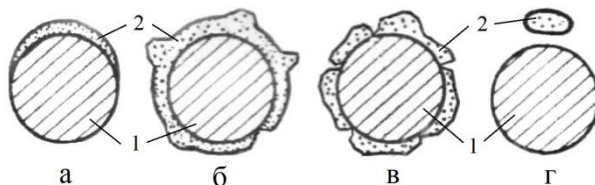
Рисунок 1 – Режими приросту гранул: а – односторонній; б – оболонковий; в – нерівномірний з тріщинами; г – з утворенням нових центрів грануляції; 1 – мінеральна гранула; 2 – суха органічна речовина.
