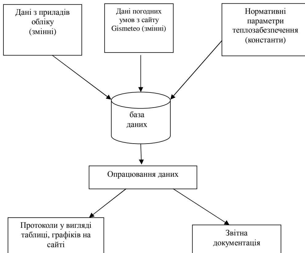
Рис .3. Схема функціонування системи моніторингу теплоспоживання будівлями СумДУ
