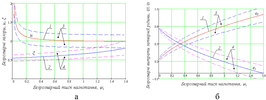
Рисунок 1 – Статичні (а) і витратні (б) характеристики запірно-урівноважуючого пристрою ротора багатоступінчатого відцентрового насоса: 1, 2 – математичні очікування; 3, 4 – довірчі області
