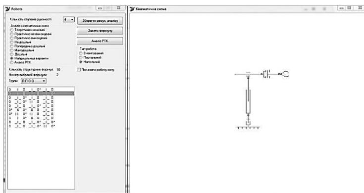
Рисунок – Інтерфейс програмного середовища для аналізу кінематичних схем промислових роботів
