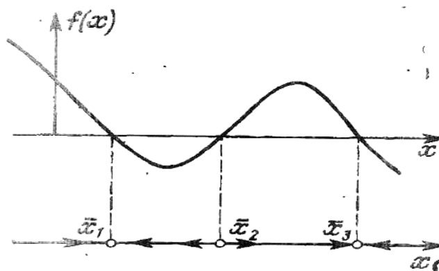
Фазова пряма
