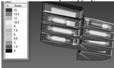
Рис. 2 – Комп'ютерне моделювання гідродинамічних процесів у шнековому вхідному пристрої (FlowVision)
