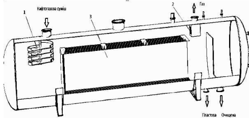
Рис. 1 – Вискоэффективный трифазный сепаратор: 1 – шнековый дефлектор, 2 – газодинамический бризковловлювач, 3 – жалюзийный блок.
