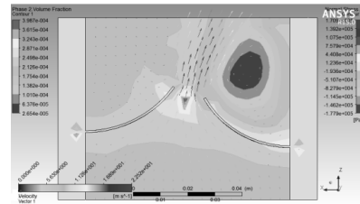
Рис. 3 – Візуалізація результатів чисельного моделювання газодинамічного брзико вловлювача (ANSYS)
