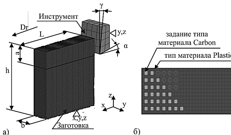
Рис. 3. Расчетная схема модели с граничными условиями и структура КЭ – сетки модели резания:
