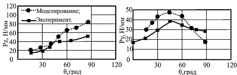
Рис. 2. Влияние угла направленности волокон на главную проекцию P_z и радиальную проекцию P_y удельной силы резания [7]
