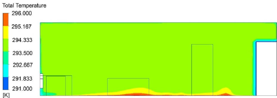
Рисунок 2.6 - Розподіл температури по висоті приміщення
