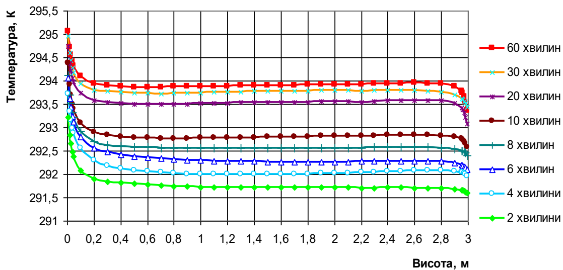
Рисунок 2.7 - Розподіл температури по висоті приміщення у часі
