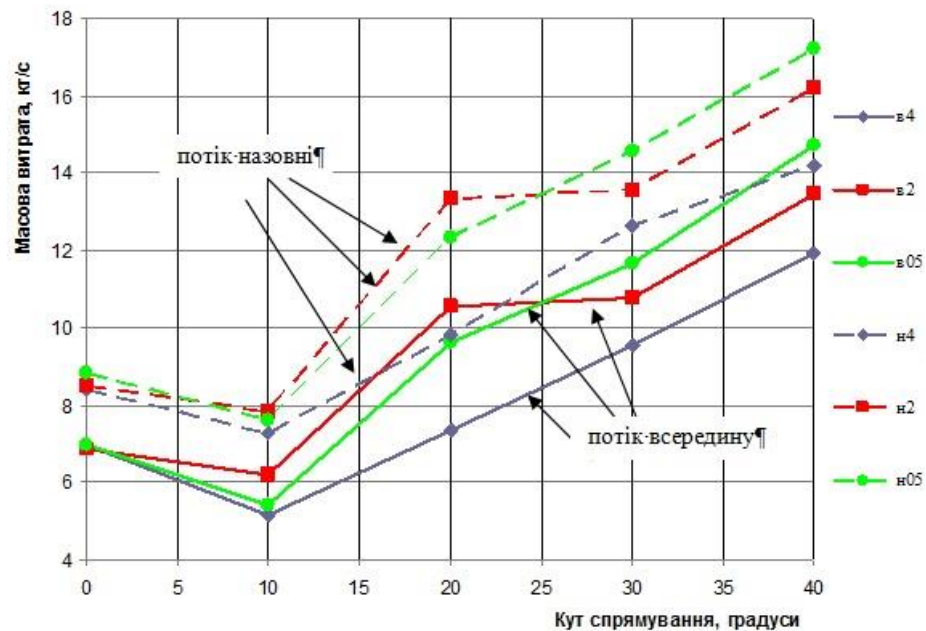
Рисунок 3.12 – Залежність кількості повітря, що витікає назовні та заходить всередину спортивного комплексу
