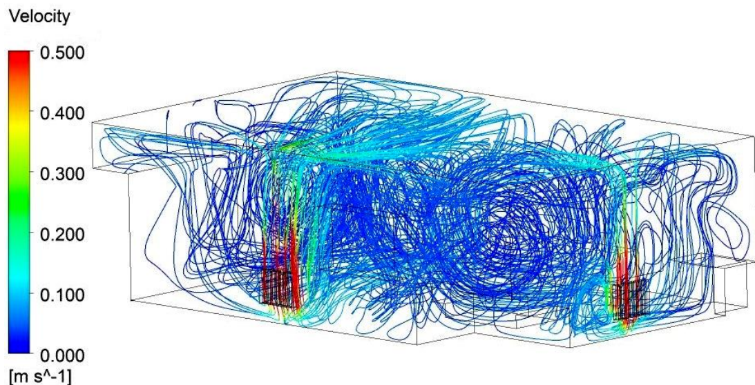
Рисунок 1.3 - Розподіл швидкостей руху повітря в об'ємі приміщення
