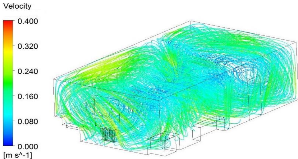
Рисунок 2.4. - Розподіл швидкостей руху повітря в об'ємі приміщення
