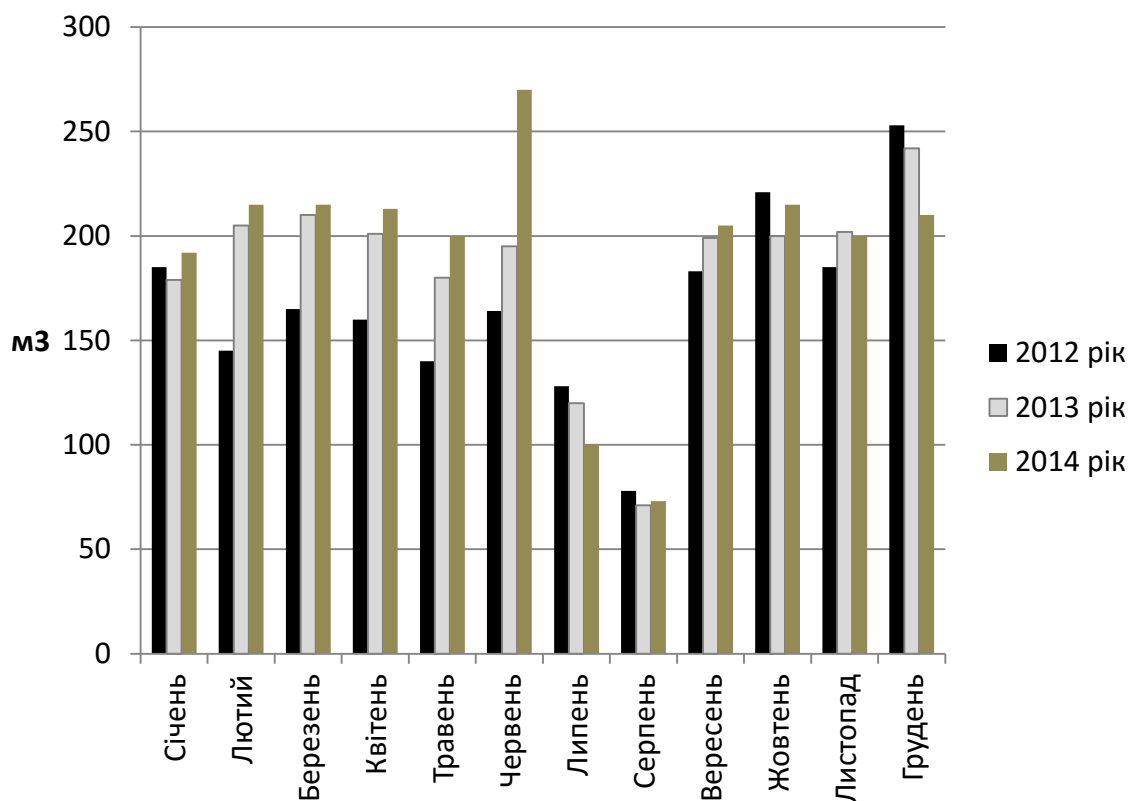
Рисунок 5.3 - Динаміка споживання холодної води навчальними корпусами у 2012, 2013 та 2014 роках
