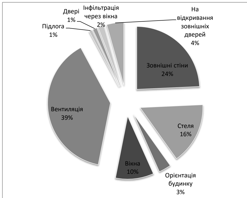
Рисунок 5.11 - Кругова діаграма розподілу основних видів тепловтрат будівлі старого корпусу «А» (центральна частина)
