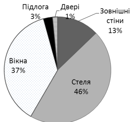
Рисунок 4.11 - Кругова діаграма розподілу основних видів тепловтрат будівлі навчального корпусу «Д».
