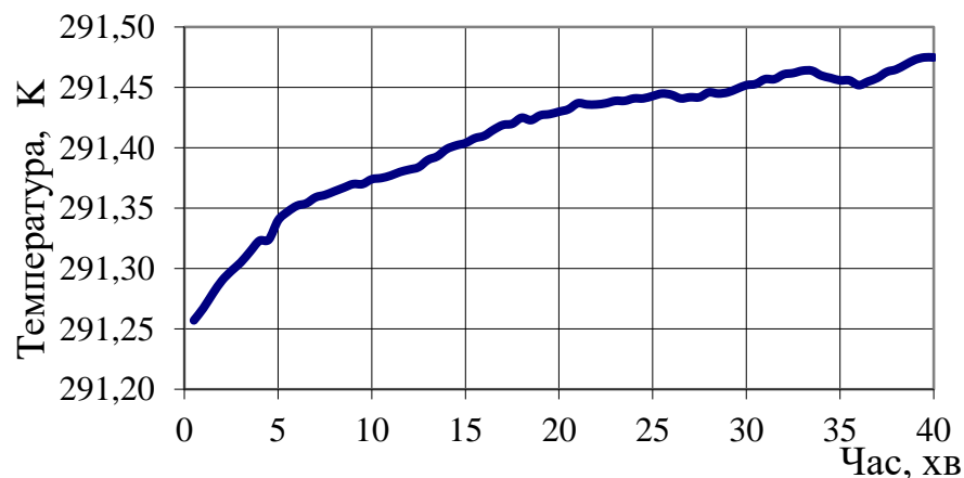
Рисунок 1. 5 Прогрівання приміщення у часі
