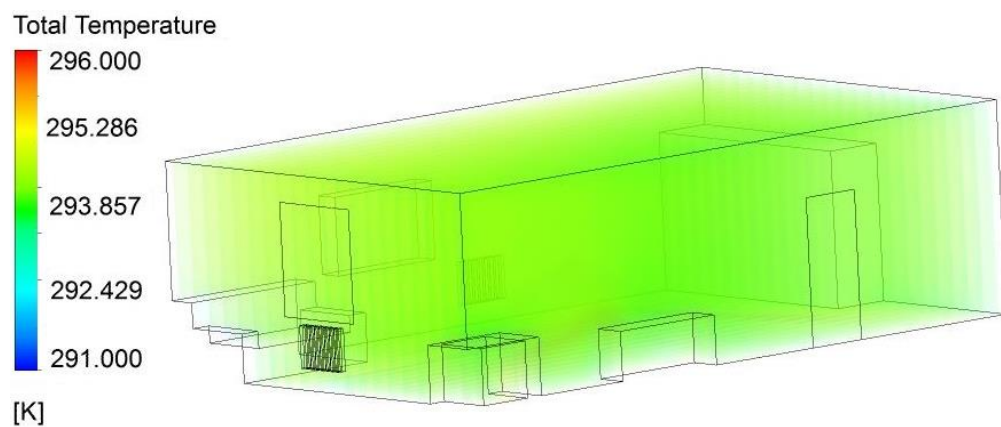
Рисунок 2.3 - Розподіл температури за об'ємом приміщення
