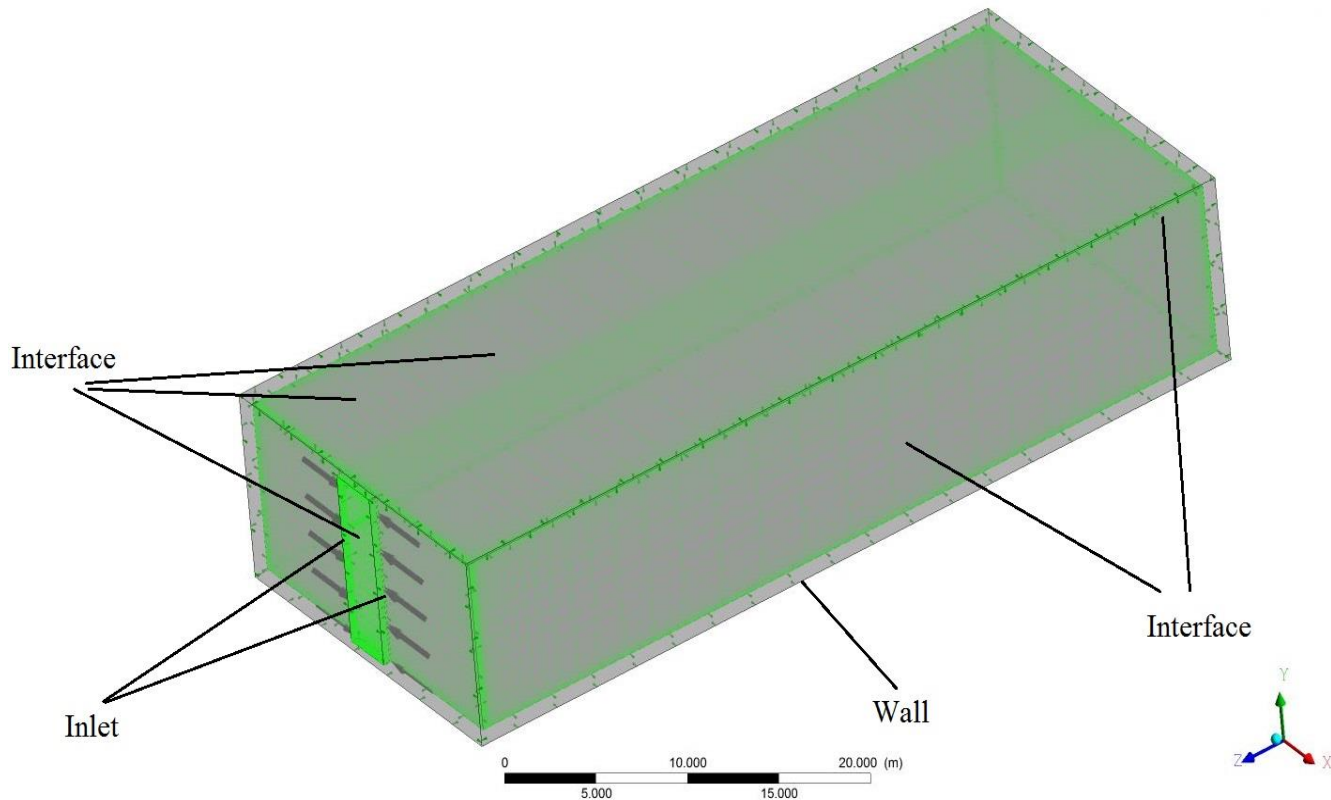
Рисунок 3.9 – Типи граничних умов для розрахункових областей Wall та Air Inside
