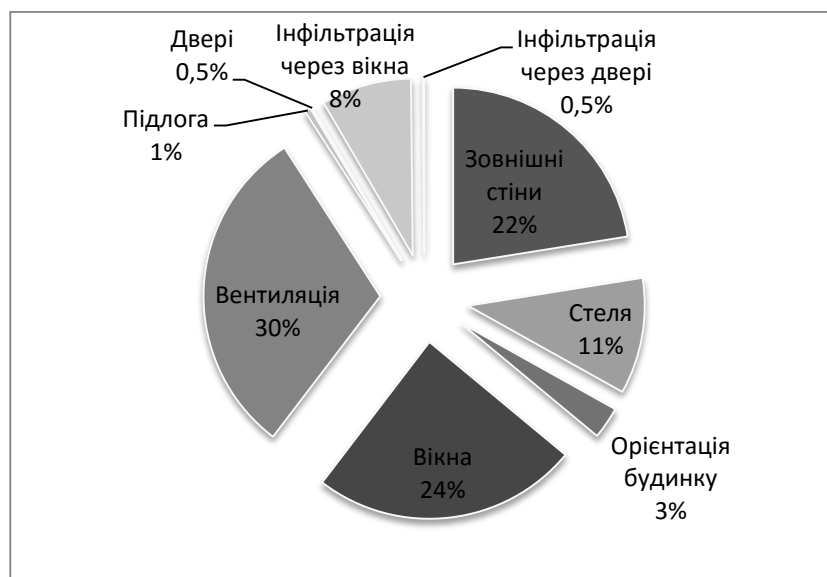
Рисунок 5.12 - Кругова діаграма розподілу основних видів тепловтрат будівлі старого корпусу «А» (навчальні приміщення)
