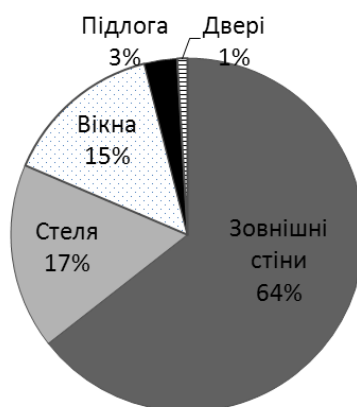
Рисунок 4.10 - Кругова діаграма розподілу основних видів тепловтрат будівлі навчального корпусу «Б».
