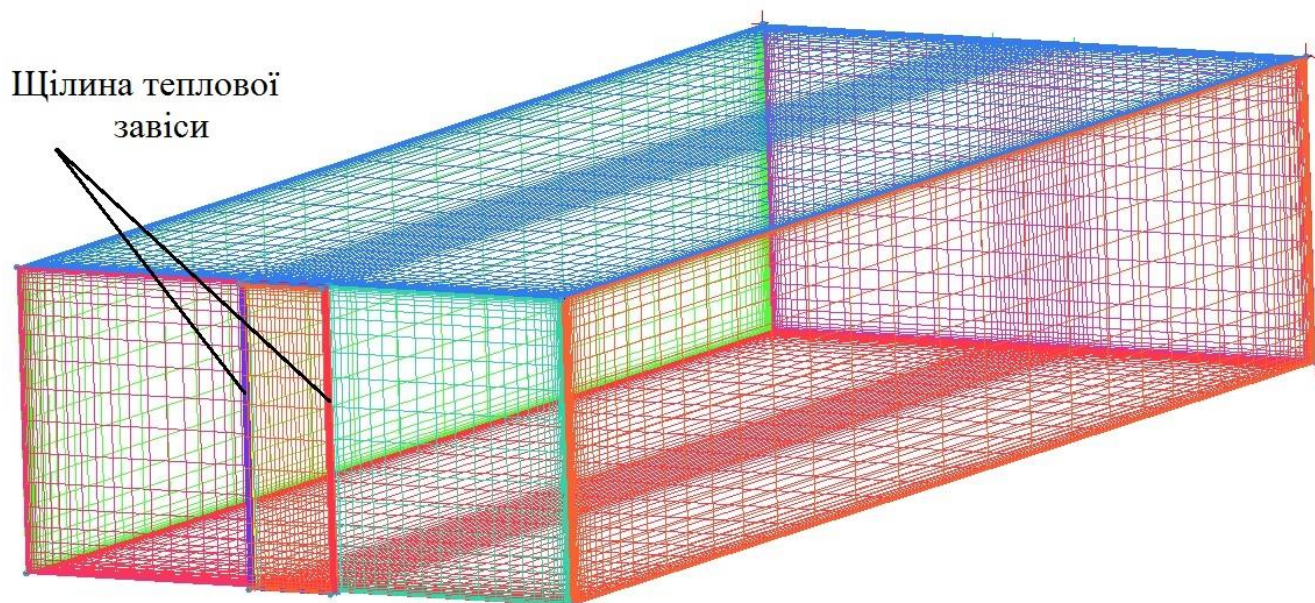
Рисунок 3.3 – Розрахункова сітка для внутрішнього повітря
