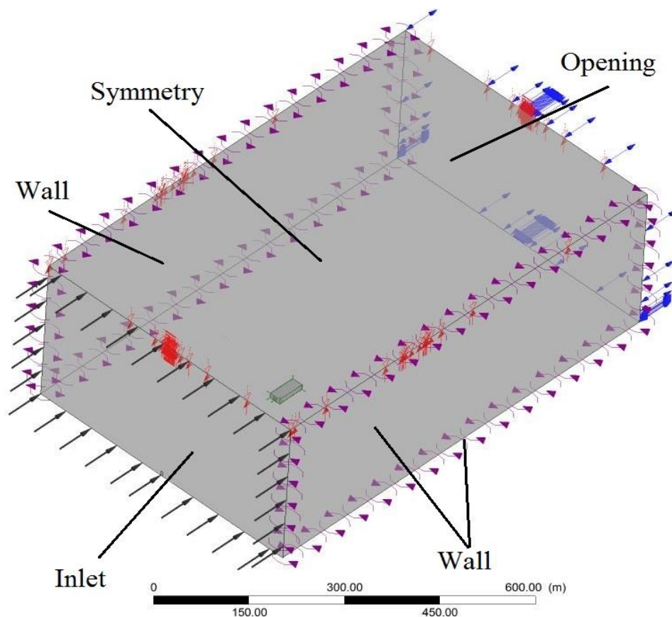
Рисунок 3.8 – Типи граничних умов для розрахункової області Inside
