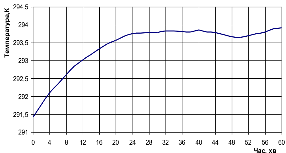
Рисунок 2.5 - Прогрівання приміщення у часі
