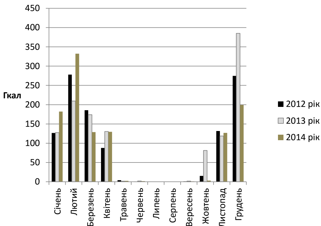
Рисунок 5.1 – Динаміка споживання теплової енергії навчальними корпусами за 2012, 2013 та 2014 роки
