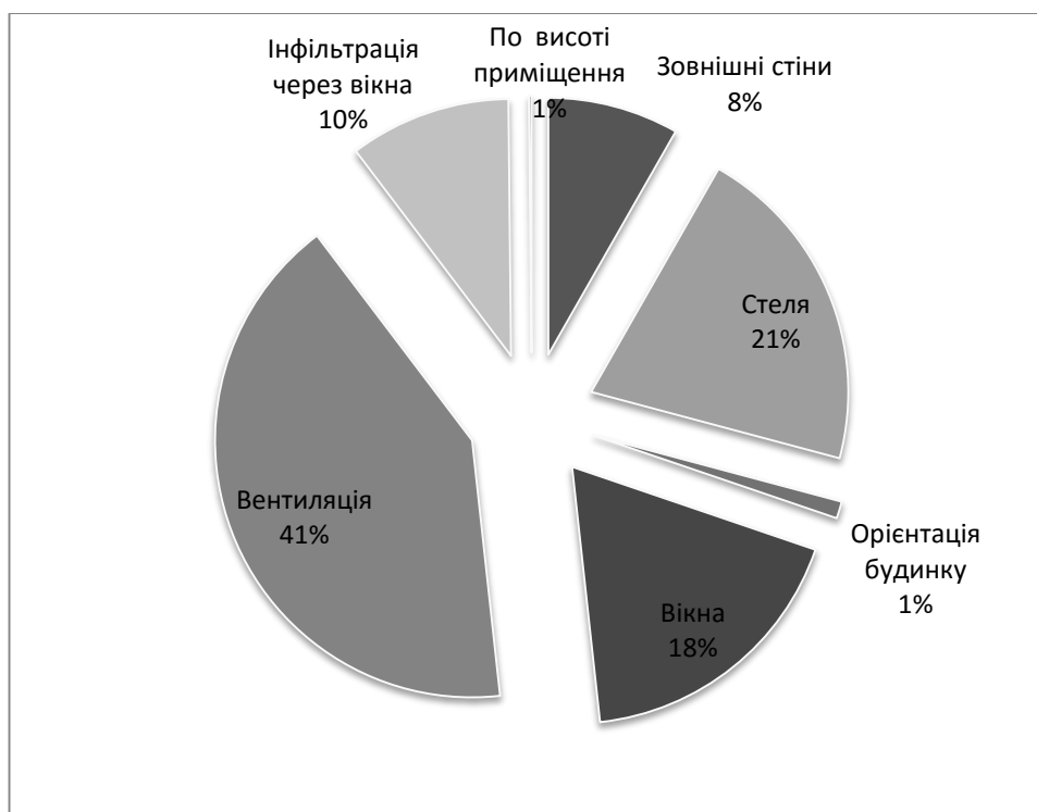
Рисунок 5.9 - Кругова діаграма розподілу основних видів тепловтрат будівлі старого корпусу «А1» (спортивна зала)
