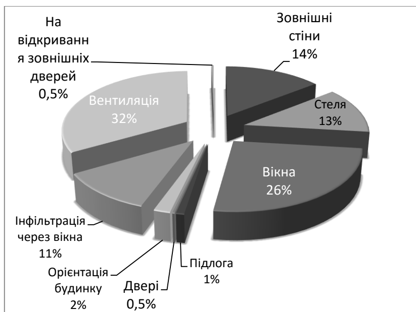
Рисунок 5.13 – Кругова діаграма розподілу тепловтрат будівлі ЗОШ №18
