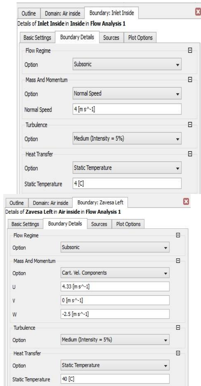
Рисунок 3.10 – Приклад задання параметрів граничних умов
