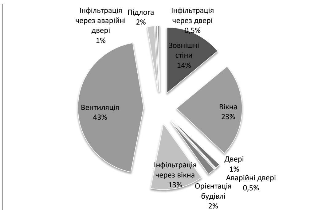
Рисунок 5.8 - Кругова діаграма розподілу основних видів тепловтрат будівлі нового корпусу «А2» (їдальня)
