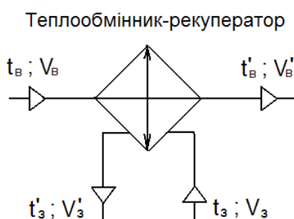
Рисунок 5.16 – Принципова схема рекуперації теплоти у системі вентиляції
