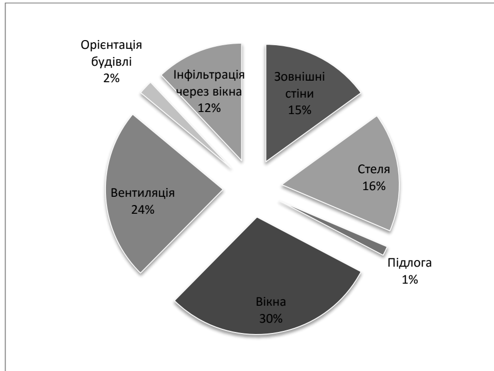
Рисунок 5.6 - Кругова діаграма розподілу основних видів тепловтрат будівлі нового корпусу «А2» (навчальні приміщення)
