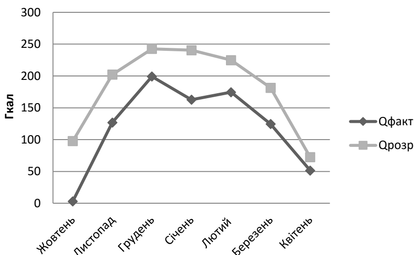
Рисунок 5.15– Співвідношення базового теплоспоживання з розрахунковим теплоспоживанням за опалювальний період 2014-2015 рр.
