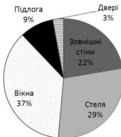
Рисунок 4.8 - Кругова діаграма розподілу основних видів тепловтрат будівлі лабораторного корпусу.
