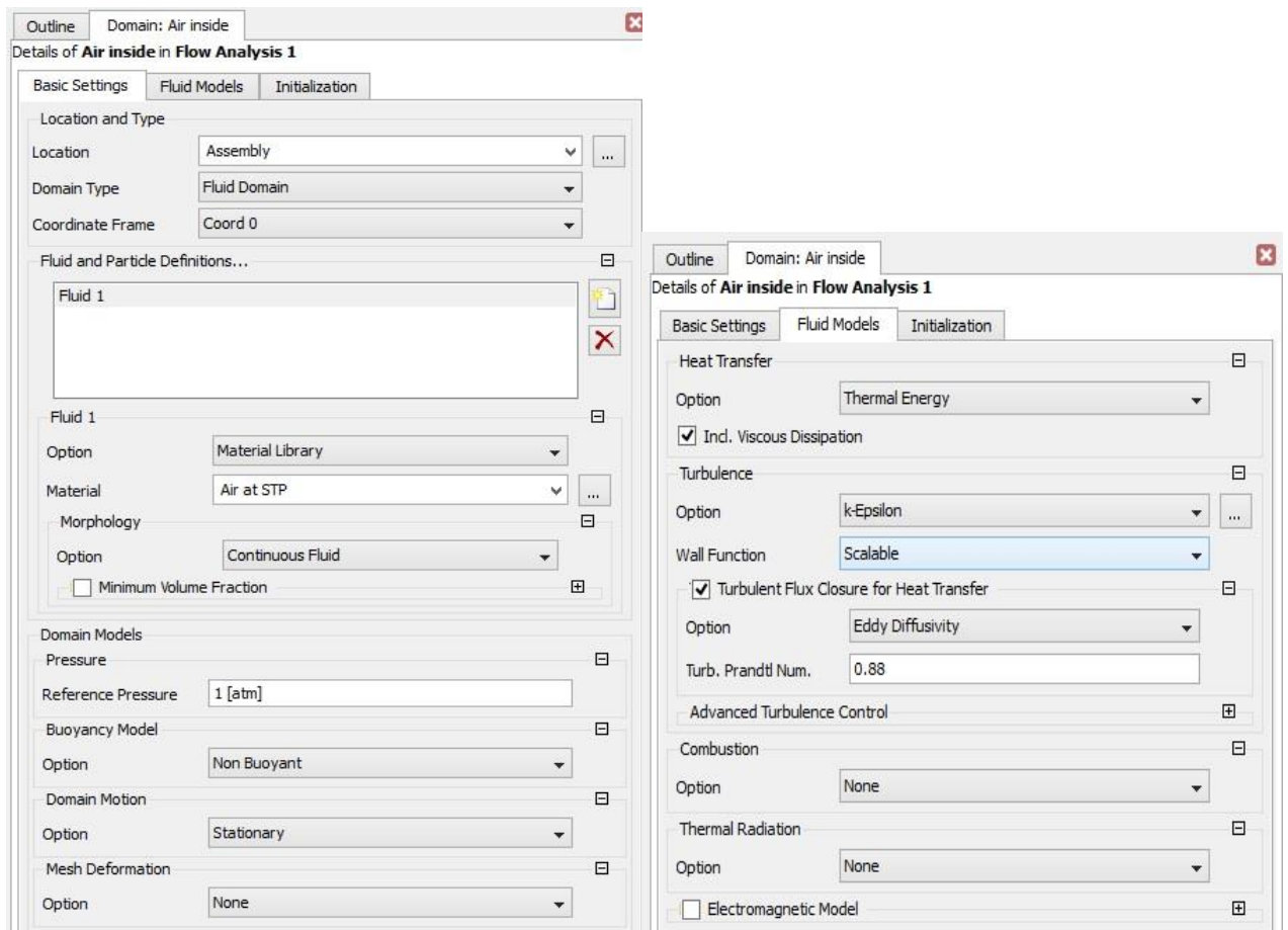
Рисунок 3.7 – Параметри робочого середовища та рідкотільної моделі
