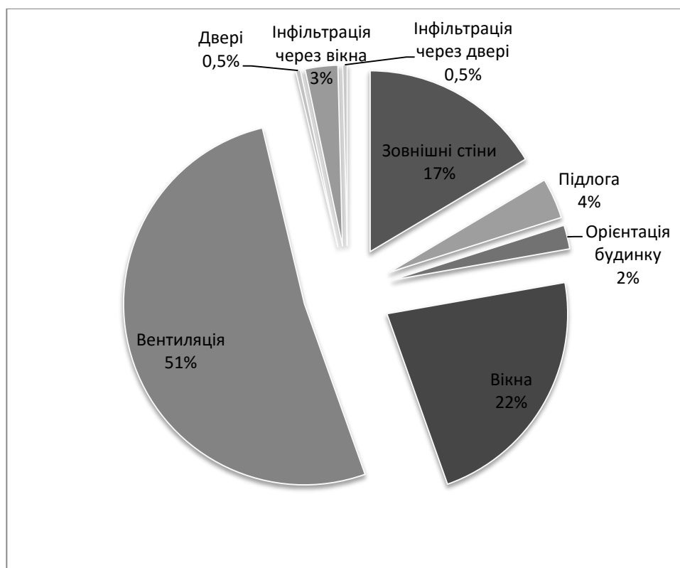
Рисунок 5.10 - Кругова діаграма розподілу основних видів тепловтрат будівлі старого корпусу «А1» (навчальні приміщення)
