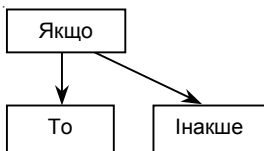
Рис. 2.8 – Схема алгоритму
