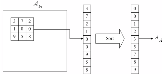
Рисунок 4 – Медианная фильтрация
