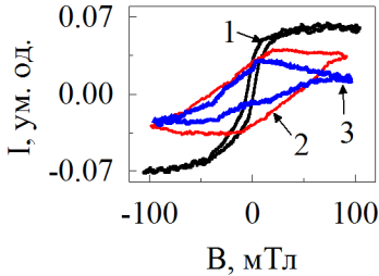
Рис. 12. Залежності МОКЕ для УМНЧ \text{Fe}_3\text{O}_4 (1), \text{CoFe}_2\text{O}_4 (2) та \text{NiFe}_2\text{O}_4 (3) після відпалу за T_6 = 1100 \text{ K}
