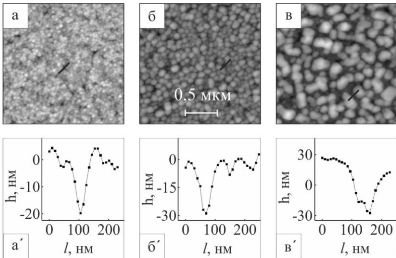
Рис. 5. Морфології поверхні зразків із товщинами ПМ \text{Ag} 5 нм (а), 10 нм (б) та 15 нм (в) після відпалювання за температури 600 К. На позиціях а', б', в' наведені відповідні профілі висоти
