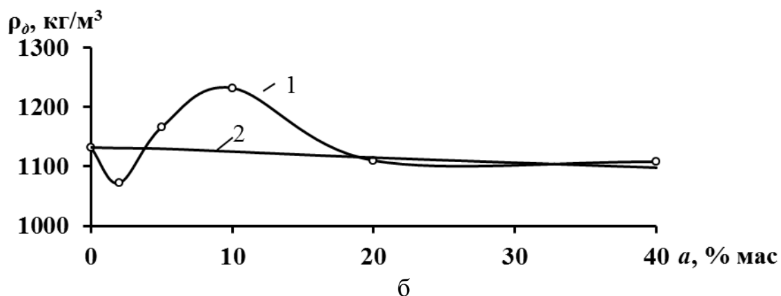
Рисунок 5.1 – Залежність щільності порохових гранул від вмісту в них камфори (а) та дибутилфталата (б)
