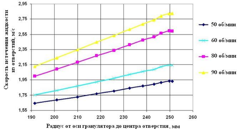
Рисунок 1.9 – Залежність швидкості витікання рідини з отворів гранулятора з 6 прямими лопатками від радіуса розташування отворів при різній швидкості обертання.
