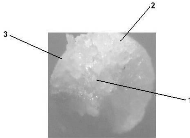
Рисунок 2.17 – Структура гранули, яку отримано за способом [27-29]: 1 – ядро гранули; 2 – перехідний шар; 3 – поверхневий пористий шар.
