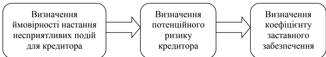
Рис. 1. Схема визначення оптимального співвідношення «кредит – застава»
