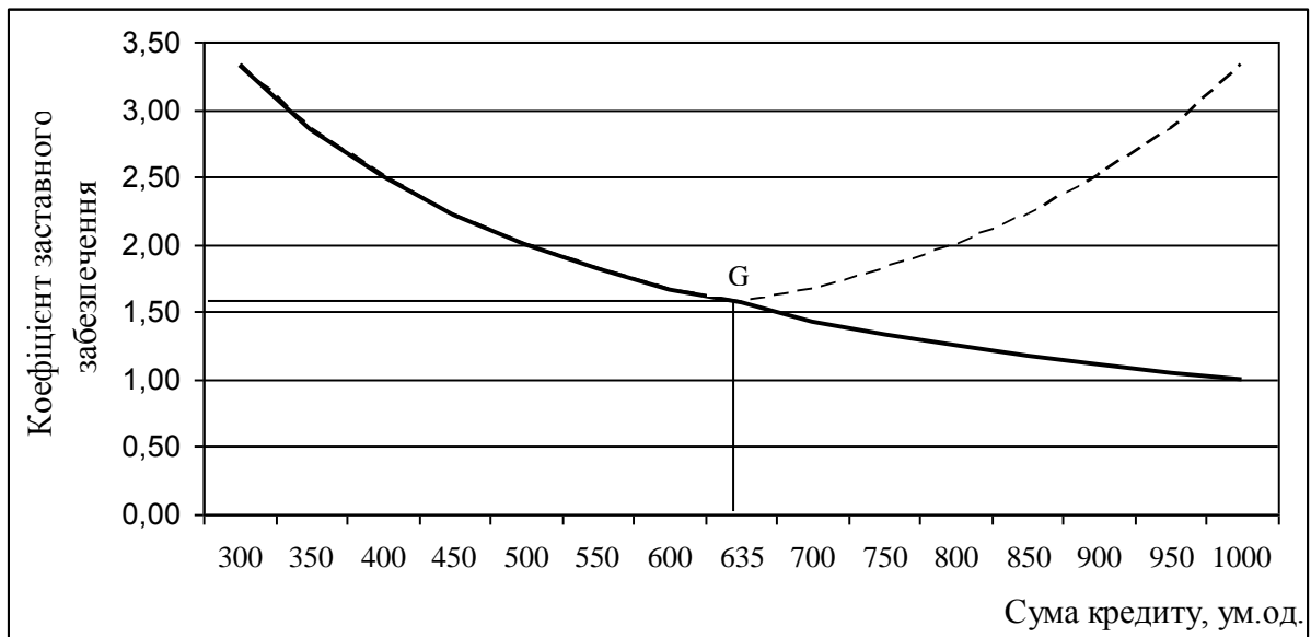
Рис. 2. – Визначення оптимального співвідношення «кредит – застава» для промисловості
