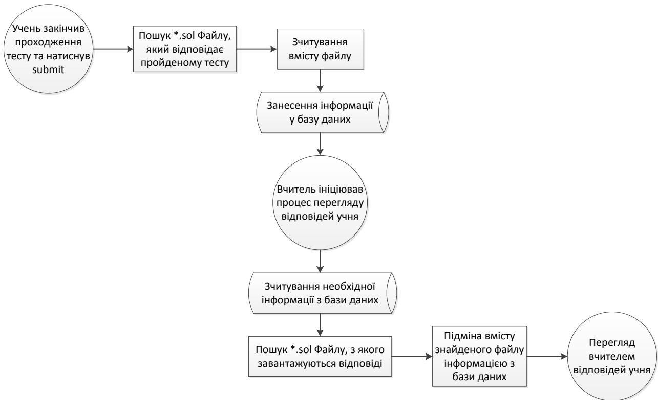
Рисунок 3 – Алгоритм рішення
