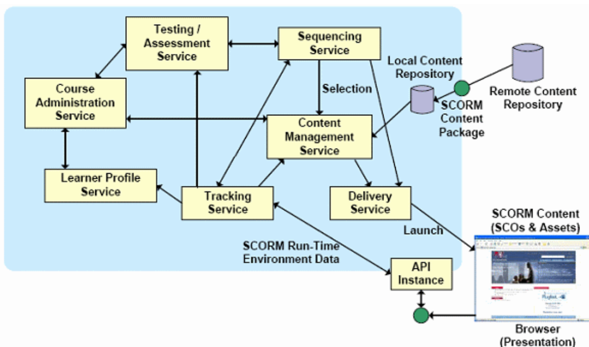
Рисунок 1 – Типова функціональна архітектура LMS
