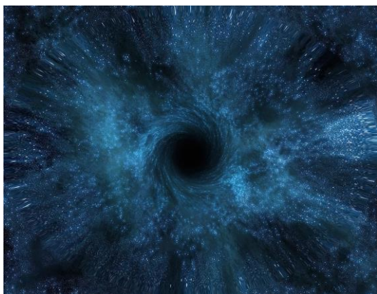
Кротова нора
