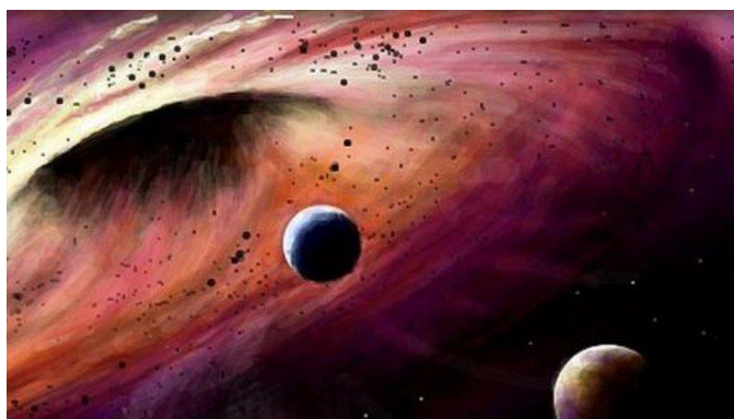
Чорна діра
