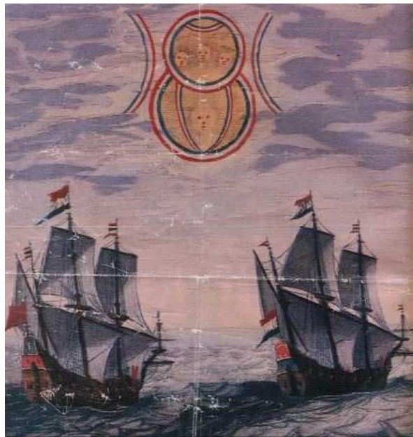
Я. В. Блау (1596–1673). НЛО над голландськими суднами. Географічний атлас (1630-і)
