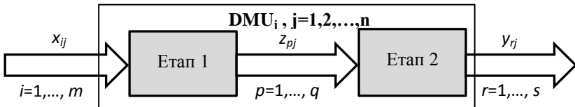
Рис. 1. Схема двокрокового методу DEA
