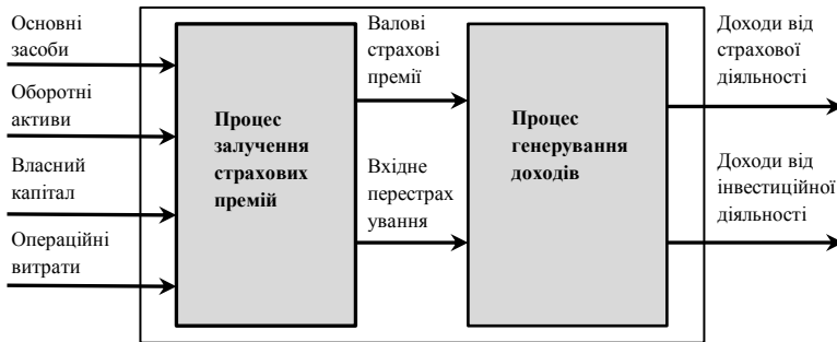
Рис. 2. Двокрокова модель оцінки ефективності СК
