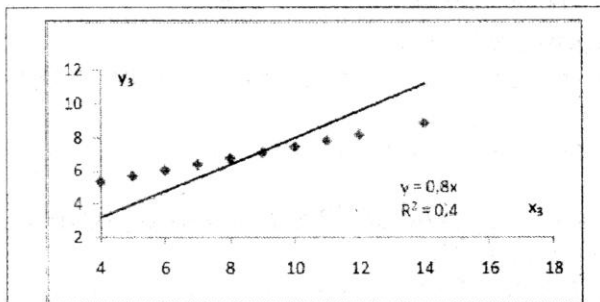
Рис. 3. Графік 3-го набору даних
