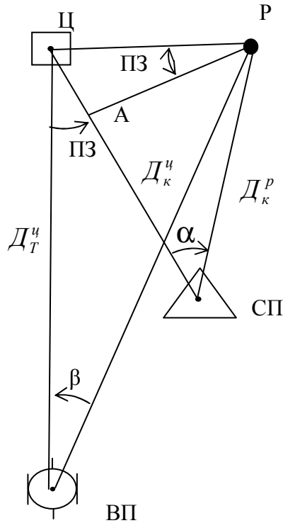
Рисунок 6.1 – Коефіцієнт віддалення
