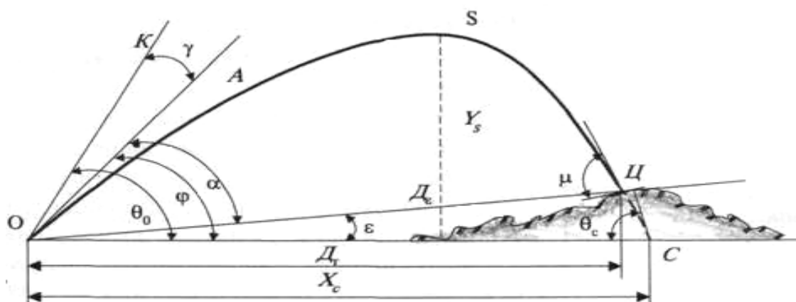
Рисунок 2.1 – Елементи траєкторії
