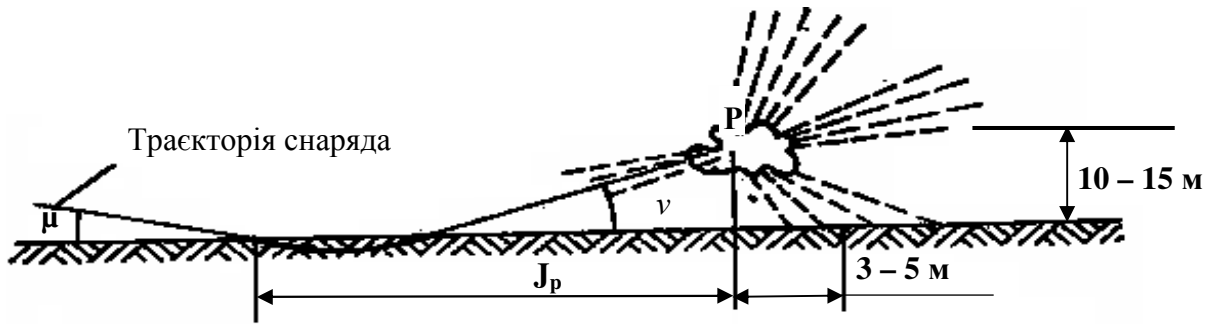
Рисунок 7.5 – Явище рикошету
