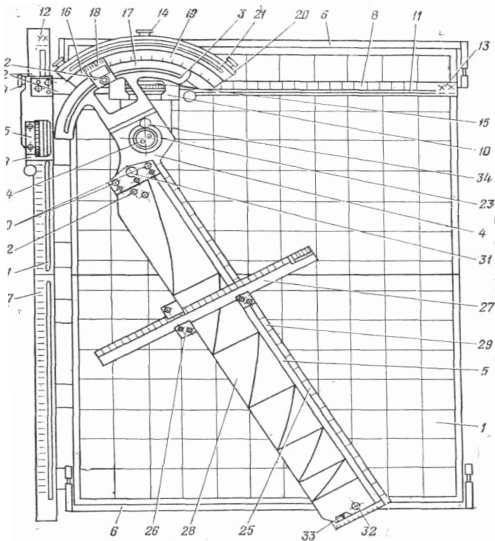
Рисунок 5.7 – Загальний вигляд приладу ПУВ-9:
