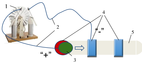
Рис. 1. Модель лінійного прискорювача елементарних частинок: 1 - генератор Вімшурета; 2 - з'єднувальні провідники; 3 – кулька; 4 – алюмінієва фольга; 5 – скляна трубка
