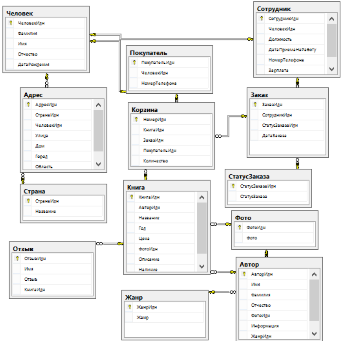
Рисунок В.1 – Діаграма зв'язків між базовими таблицями
