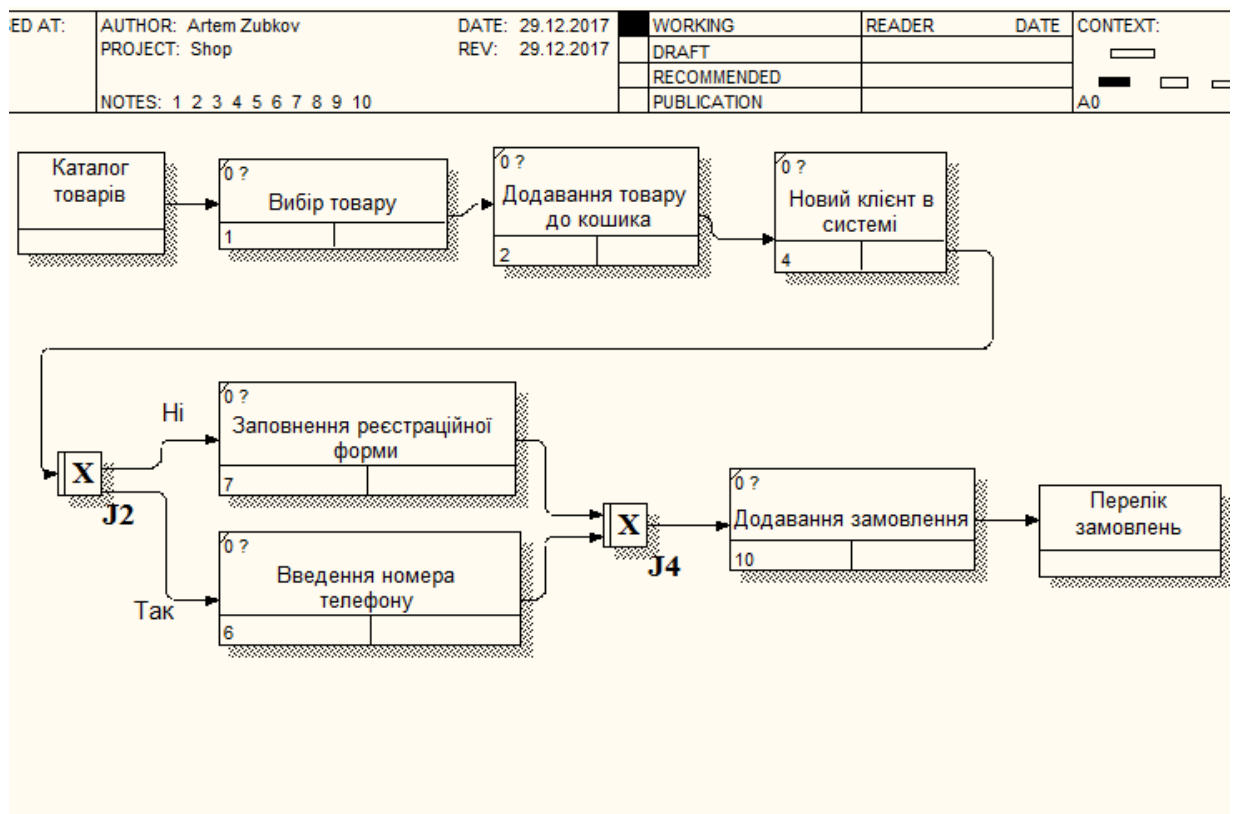
Рисунок 2.3 - Декомпозиція функціонального блоку «Замовлення товару клієнтом»
