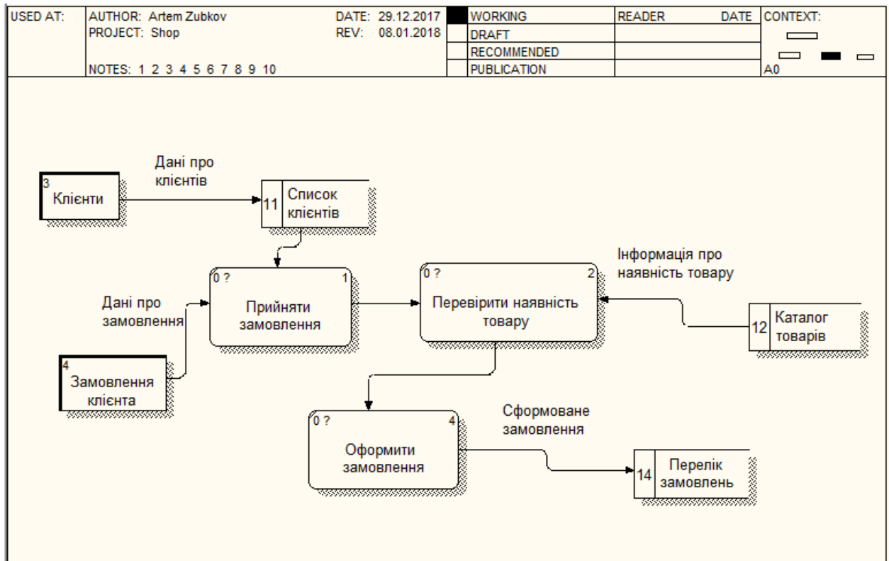
Рисунок 2.4 - Декомпозиція процесу «Оформлення замовлення»
