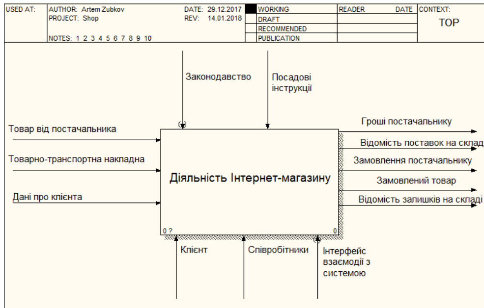
Рисунок 2.1 – Контексна діаграма «Діяльність Інтернет-магазину»
