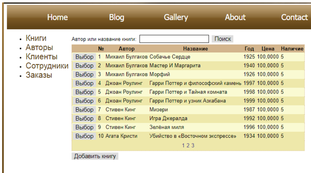
Рисунок 3.5 – Сторінка «Книги»
