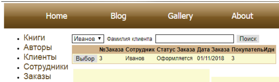
Рисунок 3.15 – Сторінка «Заказы»
