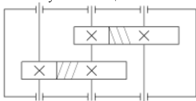
Рисунок 1 - Кинематическая схема двухступенчатого цилиндрического зубчатого редуктора
