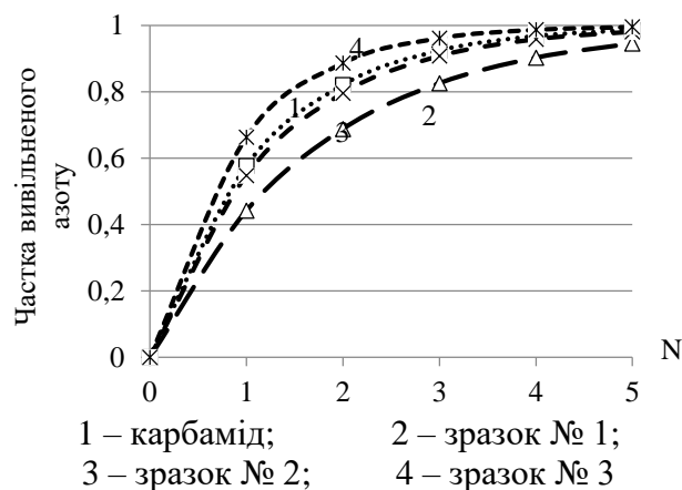
Рисунок 12 – Уніфікована крива вивільнення азоту із ґрунту під час розчинення добрив
