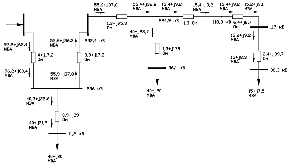
Расчетная схема замещения сети в аварийном режиме работы
