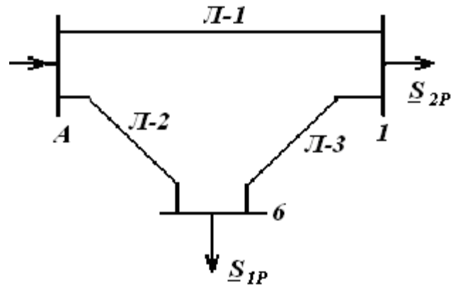
Малюнок 2 Замкнута мережа
