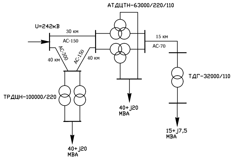
Исходная схема заданной сети
