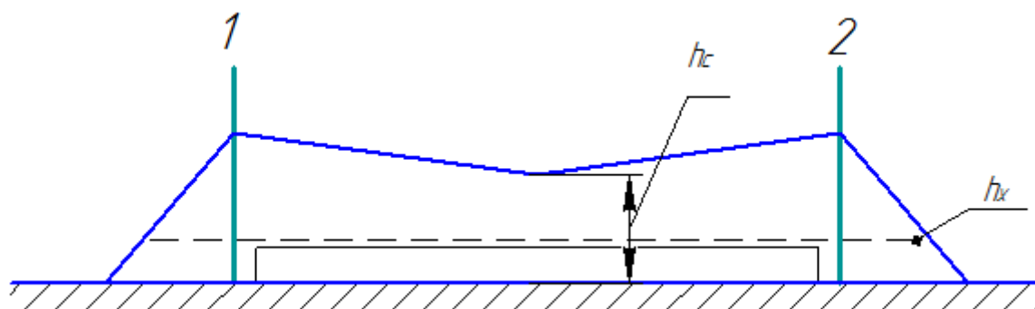
Рисунок 4 – Горизонтальний переріз зони захисту блискавковідводів Масштаб 1:1000 мм
