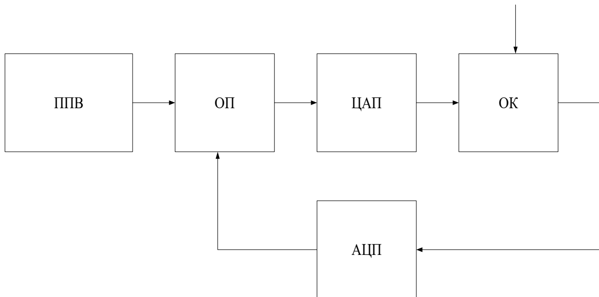
Рисунок 3.2 - Цифрова система автоматичного керування
