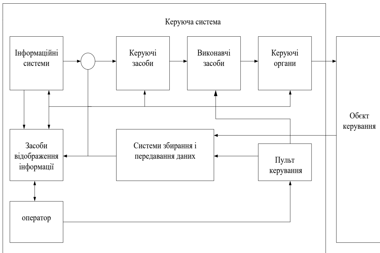
Рисунок 3.1 – Структура системи управління
