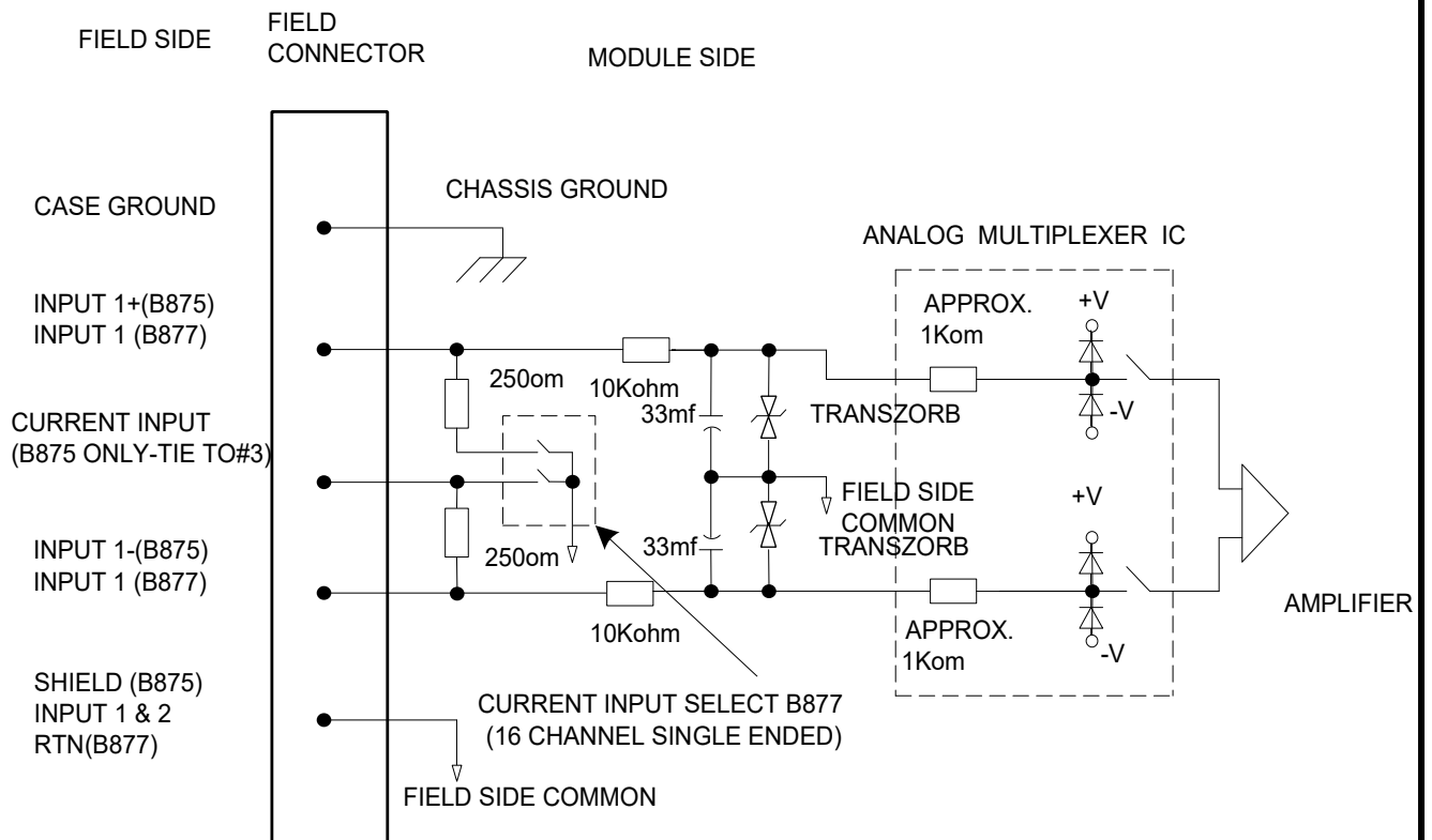
Рисунок 2.7- Схема аналого-цифрового модуля вводу Modicon B875-111
