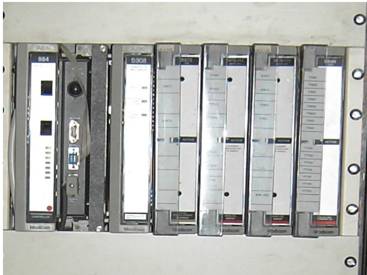
Рисунок 2.1 - Зовнішній вигляд ПЛК MODICON 984
