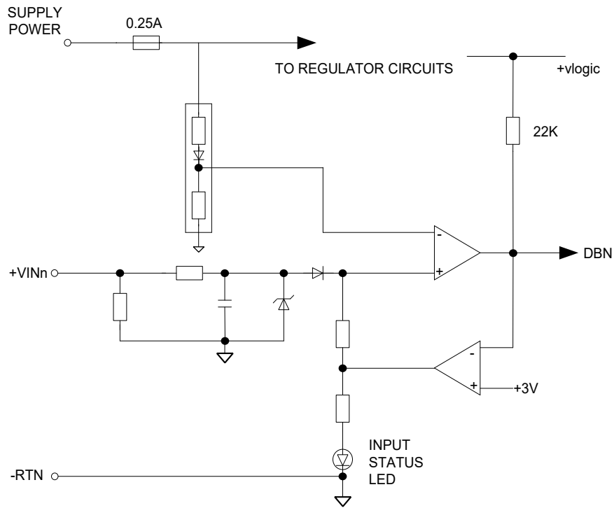
Рисунок 2.5 - Блок схема модуля вводу (Input Module) Modicon B827-032
