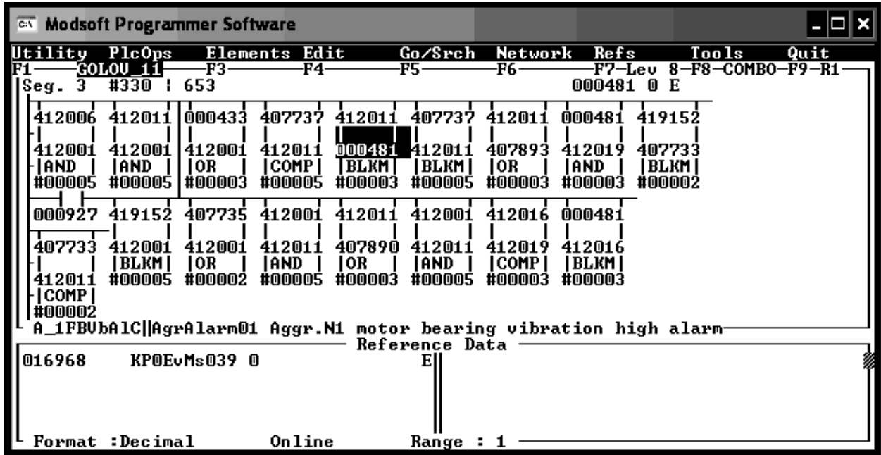
Рисунок 5.1 - Алгоритм контролю агрегатного параметра «Підвищений рівень вібрації МН»
