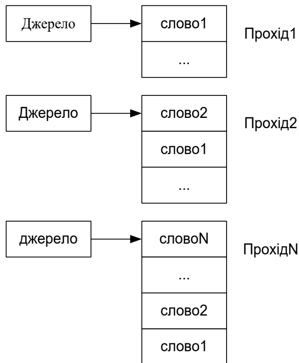
Рисунок 3.7 - Стек
