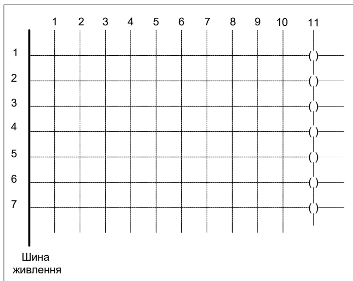
Рисунок 3.3 - Схема ступеневої логіки (Ladder Logic)
