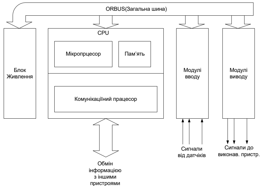
Рисунок 2.3 – Узагальнена структура ПЛК
