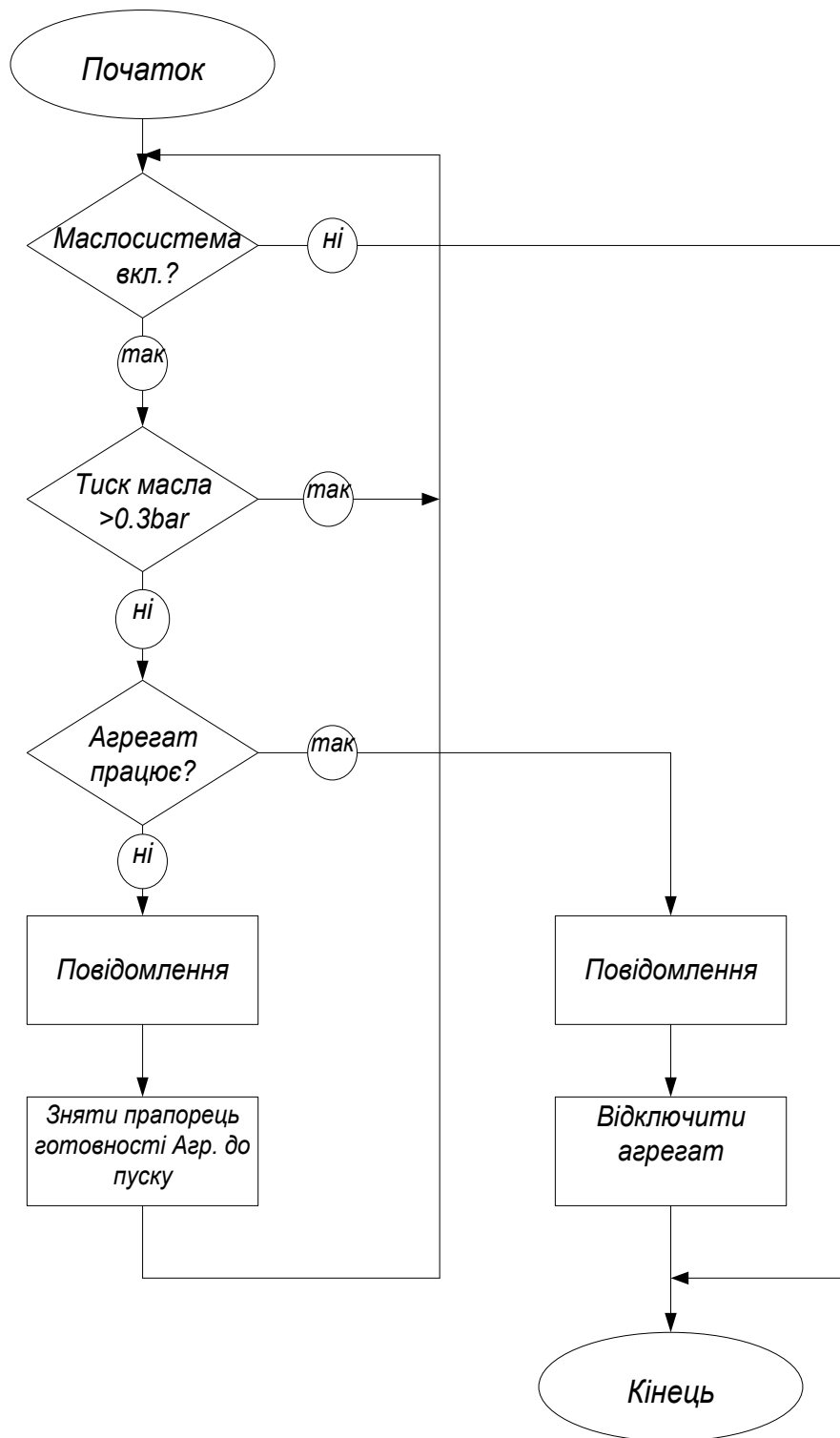
Рисунок 5.2 - Алгоритм контролю агрегатного параметра «Мінімальний тиск оливи на підшипниках МН»
