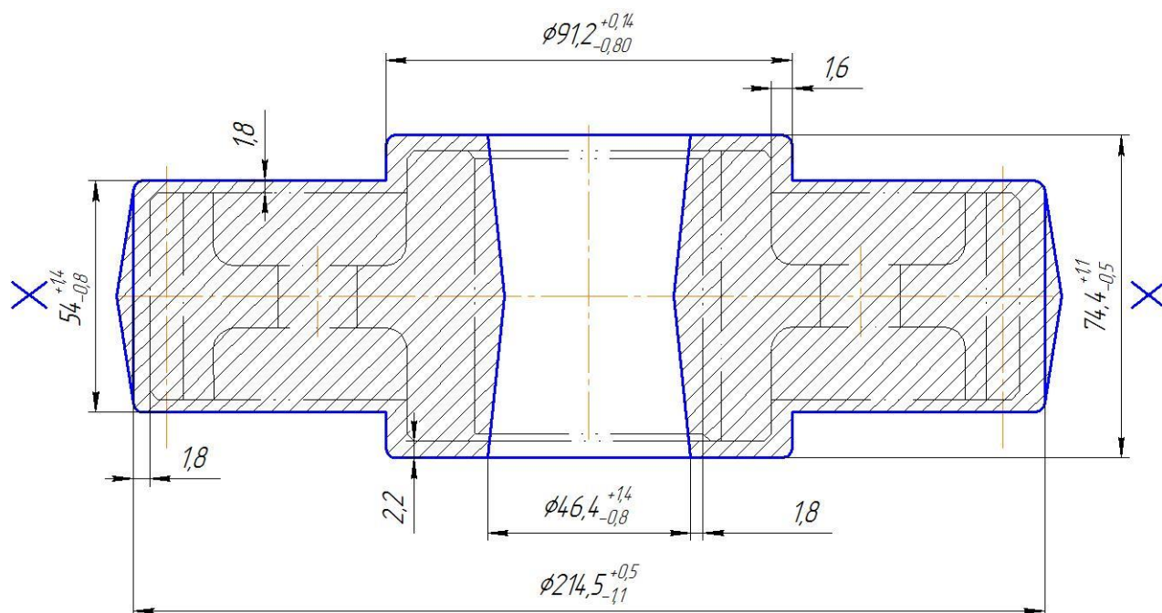
Рисунок 5.1– Ескіз штамповки
