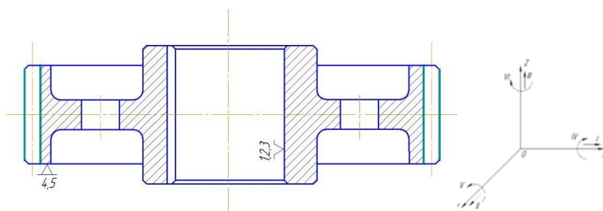
Рисунок 6.3 – Схема базування заготовки при зубонарізанні
