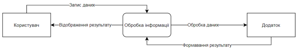
Рис. 2.2. DFD 0 діаграма
