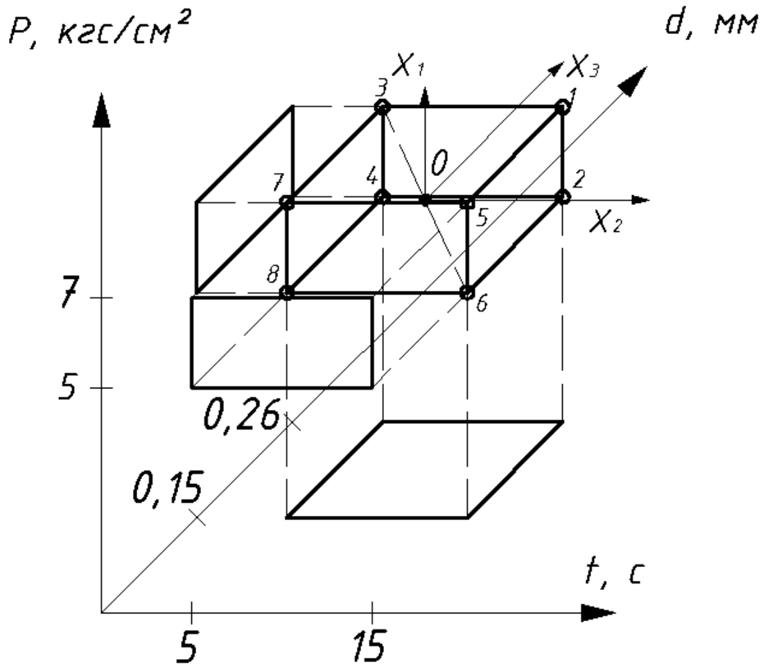
Малюнок 3.8 – Графічна інтерпретація факторного простору з граничними точками (1...8) області експериментування.
