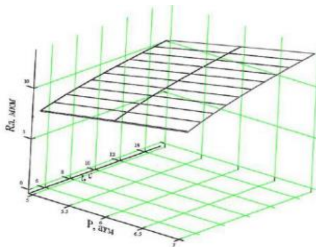
Малюнок 3.10 – Поверхня відгуку при абразивоструменевому обробленні абразивом з середнім розміром фракційного складу d_{\text{абраз}} = 0,2 мм
