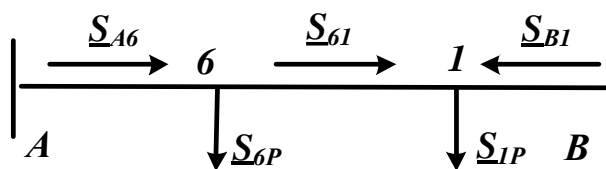
Рисунок 1.3 – Разімкнута мережа
