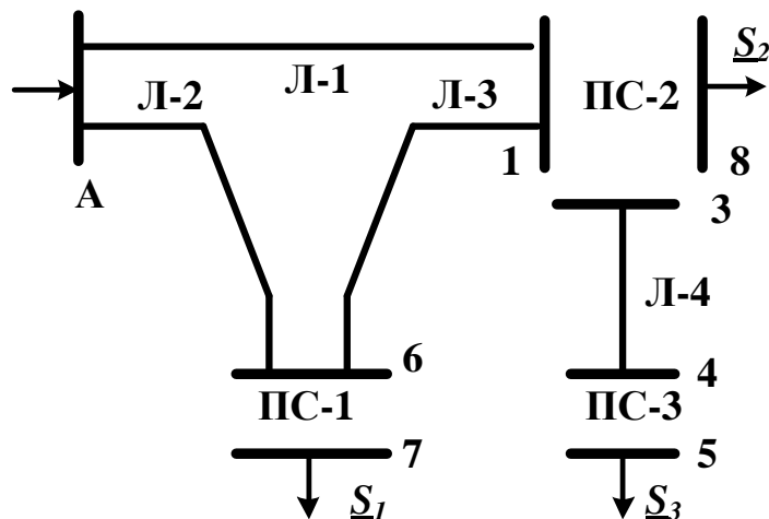
Рисунок 1.1 – Однолінійна електрична схема заданої електричної мережі
