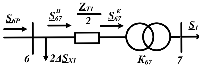
Рисунок 1.4 – Схема заміщення підстанції ПС-1
