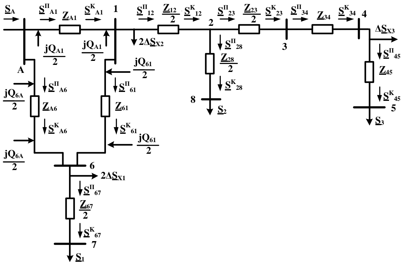
Рисунок 1.9 – Повна схема заміщення мережі
