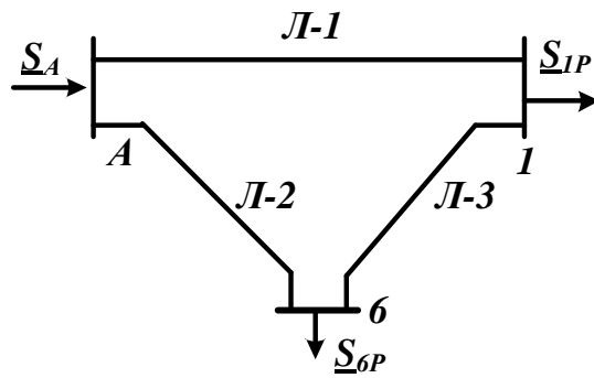
Рисунок 1.2 – Замкнута мережа
