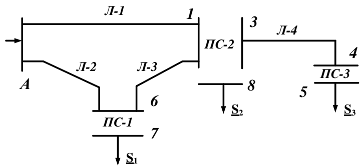
Початкова схема мережі
