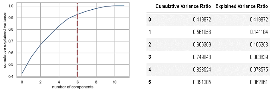
Рисунок 2 – Результати застосування методу головних компонент (розраховано авторами самостійно)
