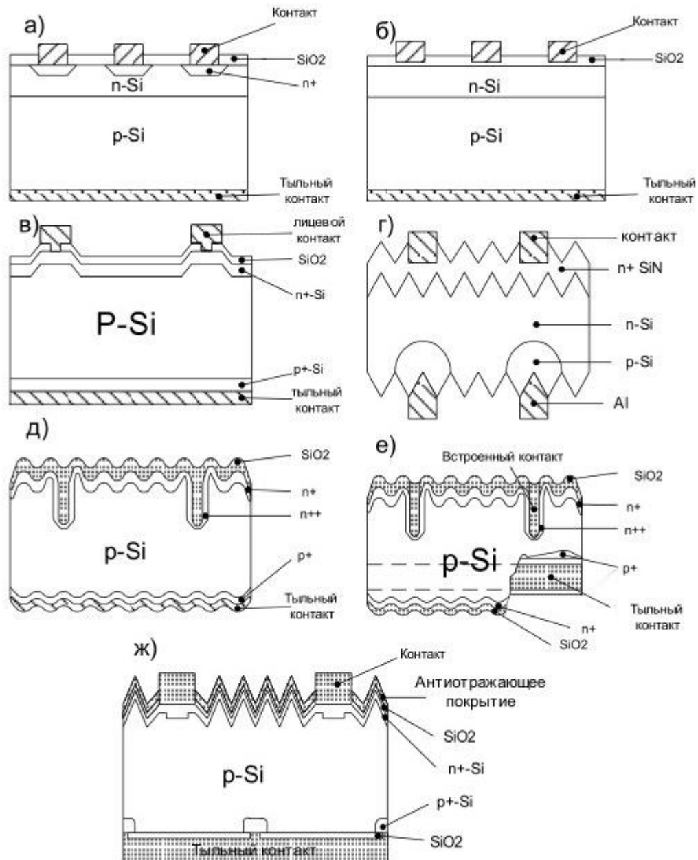
Рис.2.1.Різні типи СЕ на основі монокристалічного кремнію. а – звичайний p-n перехід; б – структура метал-ізолятор; в – СЕ з пасивованим емітером; г – двосторонній СЕ; д – структура з одностороннім вбудованим контактом; е – структура з двостороннім вбудованим контактом; ж – структура з пасивованим емітером та локально-дифузійним вбудованим контактом [21]
