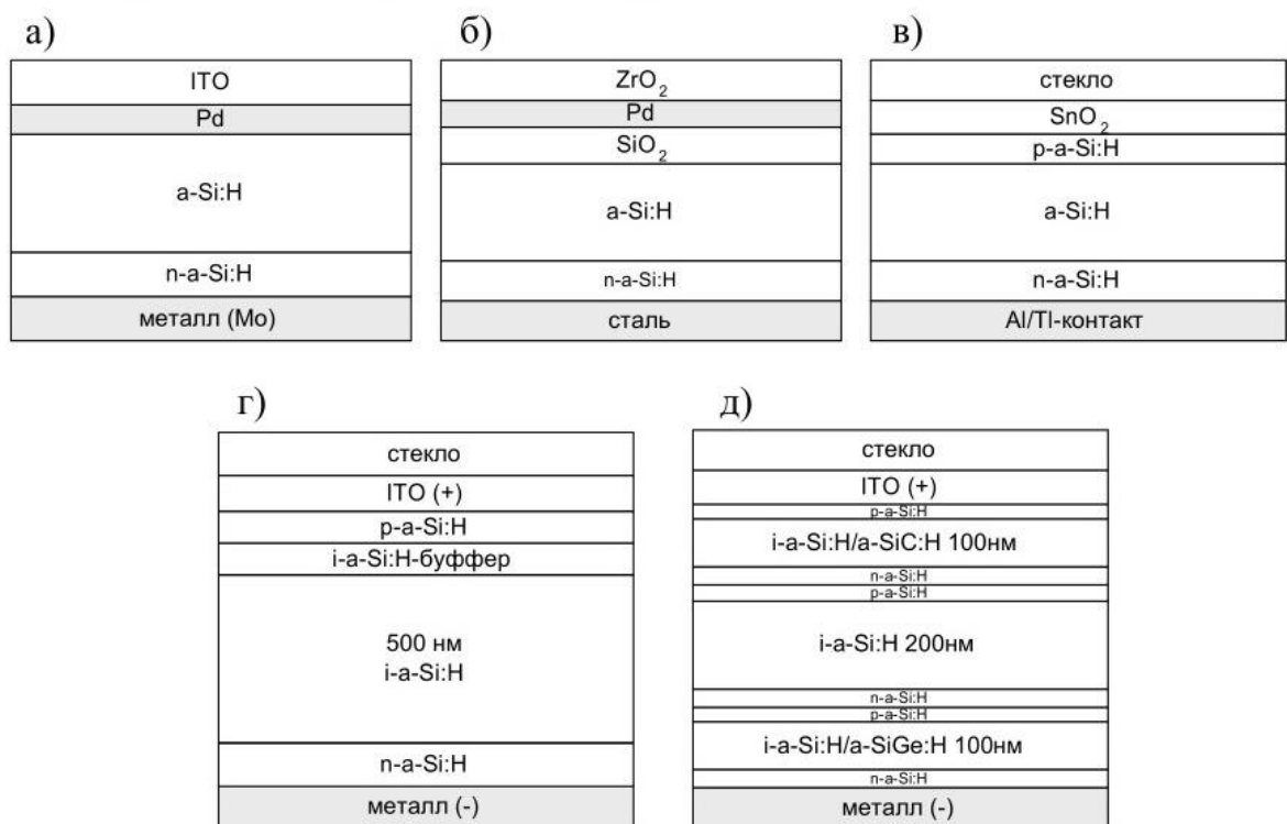
Рис. 2.2. СЕ на основі аморфного кремнію: а – бар'єр Шоттки; б – МДП-структура; в – p-i-n -структура; г – p-i-n -структура з буферним шаром; д – трьох перехідний елемент [21].
