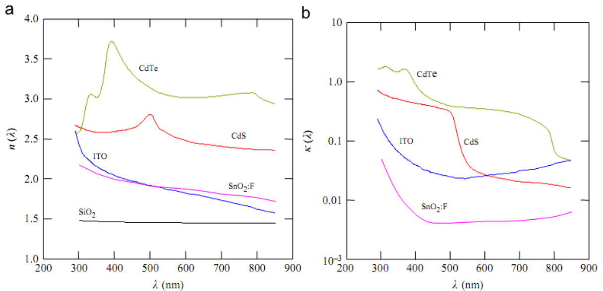
Рис. 3.1 – Показники заломлення (а) та оптичного ослаблення (б) фотоперетворювача
