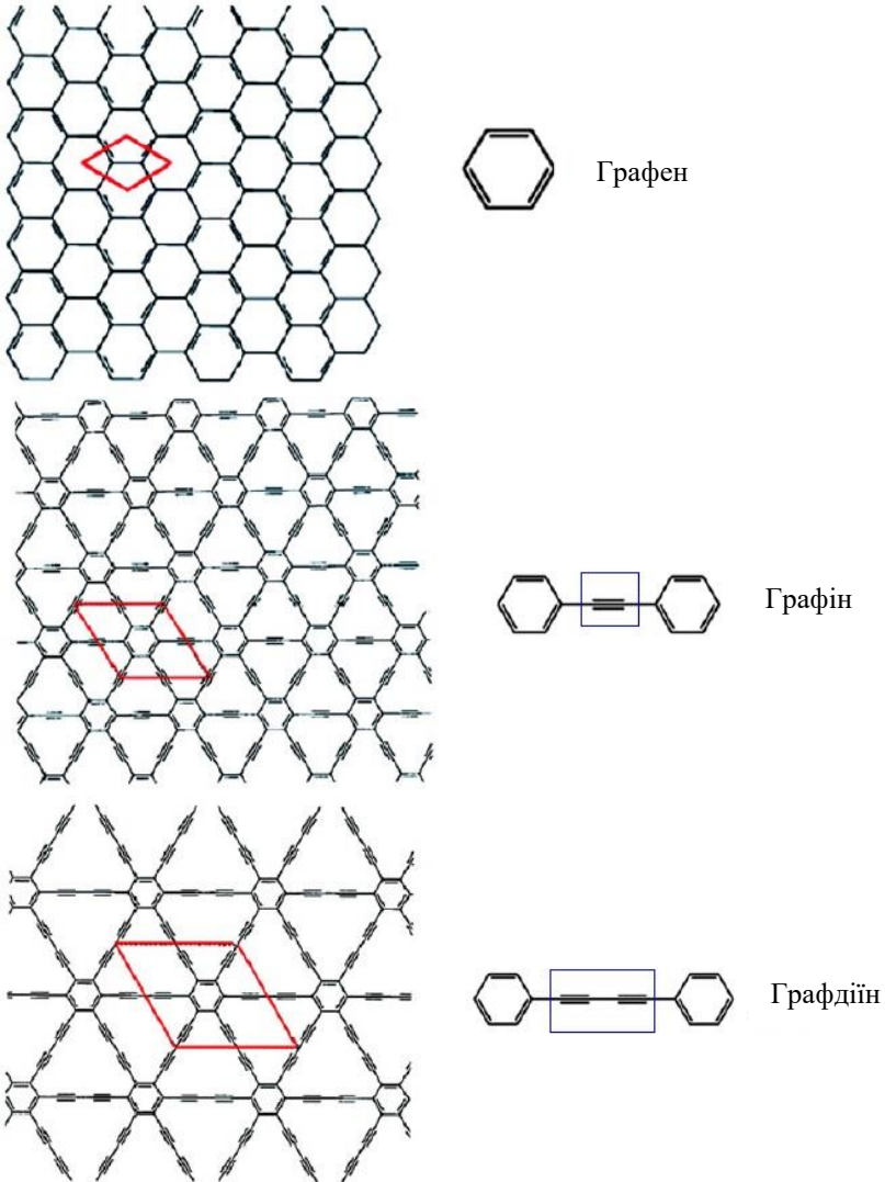
Рисунок 3.28 – Схематичні структури графену, графіну, графдіїну. Відповідні бензольні кільця, пов’язані з ацетиленовими зв’язками, показані праворуч. Червоні паралелограми є елементарними клітинками, а сині квадрати показують ацетиленові зв’язки [46]
