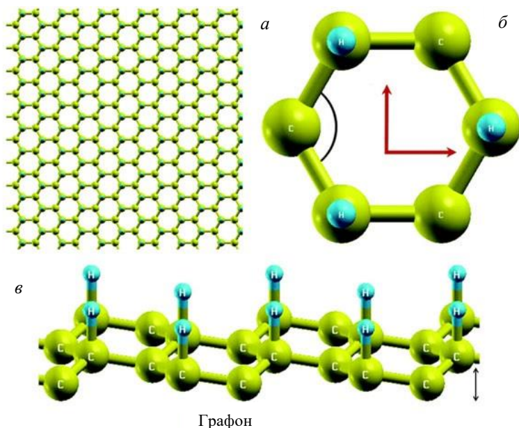
Рисунок 3.25 – Геометрія графенового листа: a – вигляд зверху; б – конфігурація комірки; в – вигляд збоку [46]
