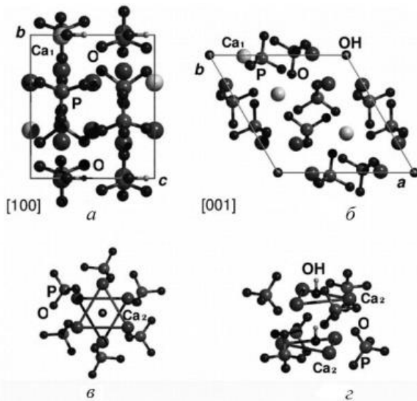
Рисунок 3.21 – Кристалографічна структура ГА: a – координаційне оточення іонів Ca_1 з урахуванням кристалографічного спрямування [100] ; б – кристалографічна структура ГА, спроектована на базову площину елементарної комірки [001] ; в – трикутники іонів Ca_2 навколо OH -каналу з оточенням із семи іонів кисню; г – проєкція [33]
