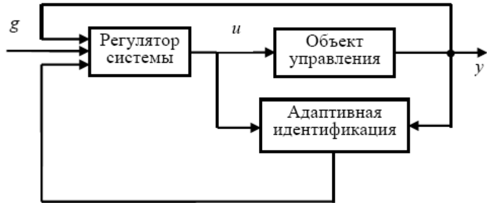
Малюнок 1 Адаптивна система управління з настроеною моделлю (АСНМ)
