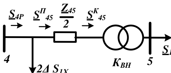
Рисунок 1.8 – Схема заміщення підстанції ПС-1
