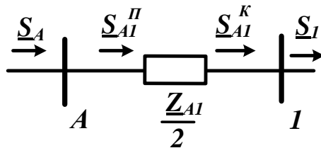
Рисунок 1.10 – Схема замещения лінії А –1
