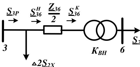
Рисунок 1.5 – Схема заміщення підстанції PC-2
