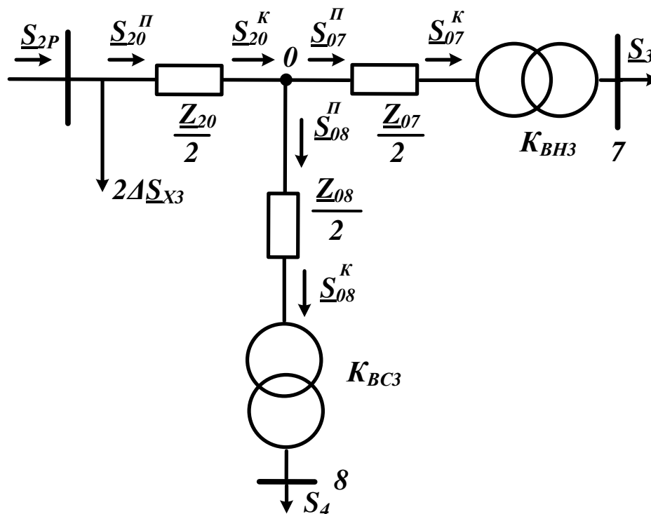
Рисунок 1.6 – Схема заміщення підстанції ПС-3
