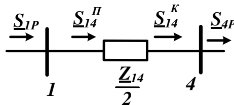
Рисунок 1.9 – Схема заміщення лінії 1–4
