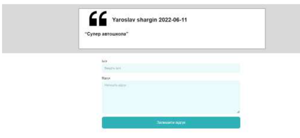
Рисунок 3.11 – Блок відгуків
