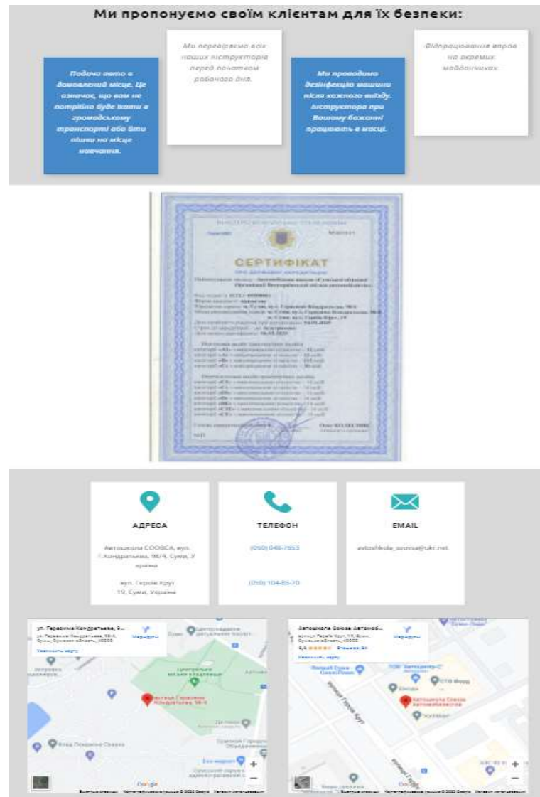
Рисунок 3.1 – Головна сторінка
