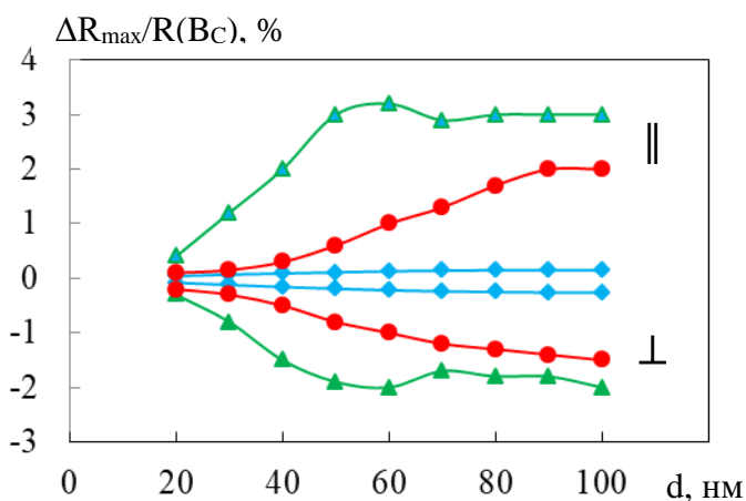
Рисунок 3.2 – Розмірна залежність повздовжнього (||) та поперечного (⊥) магнітоопору плівкових сплавів FeCo (◆), FeNi (●) та CoNi (▲)
