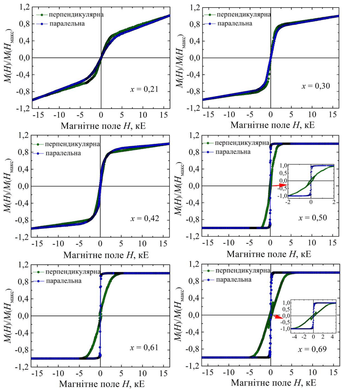
Рисунок 3.14 – Польові залежності нормованої намагніченості для невідпалених зразків плівкових сплавів на основі Ru і Cu різного складу 0,21 \leq x_{\text{Ru}} \leq 0,69 товщиною d = 40 нм, виміряні у перпендикулярній та паралельній геометріях вимірювання при T_{\text{вимір.}} = 300 К
