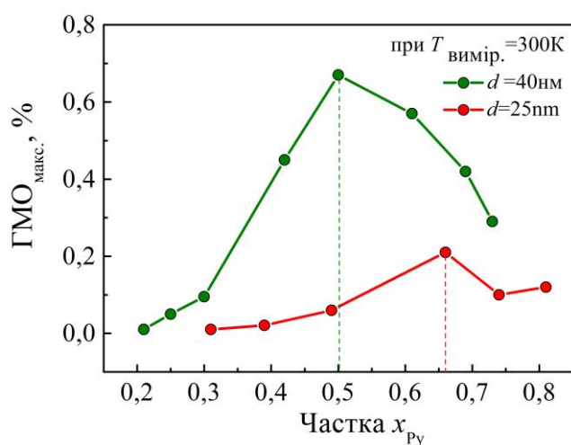
Рисунок 3.12 – Залежність величини ГМО невідпалених зразків плівкових сплавів на основі \text{Ru} і \text{Cu} товщиною 25 та 40 нм від їх складу. Вимірювання ГМО здійснювали у поздовжній геометрії вимірювання у полі H_{\text{макс}} = 4,5 \text{ кЕ} для зразків товщиною d = 25 \text{ нм} та H_{\text{макс}} = 15 \text{ кЕ} для зразків d = 40 \text{ нм} при T_{\text{вимір.}} = 300 \text{ К}
