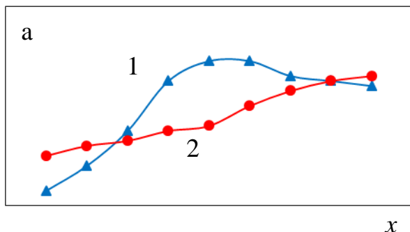
Рисунок 3.13 – Залежності значень коерцитивної сили B_C та поля насичення B_S від вмісту Fe x для плівкових сплавів \text{Fe}_x\text{Co}_{1-x}/\text{П} (криві 1) та (\text{Fe}_x\text{Co}_{1-x})_{0,5}\text{Cu}_{0,5}/\text{П} (криві 2) товщиною d=30 нм.
