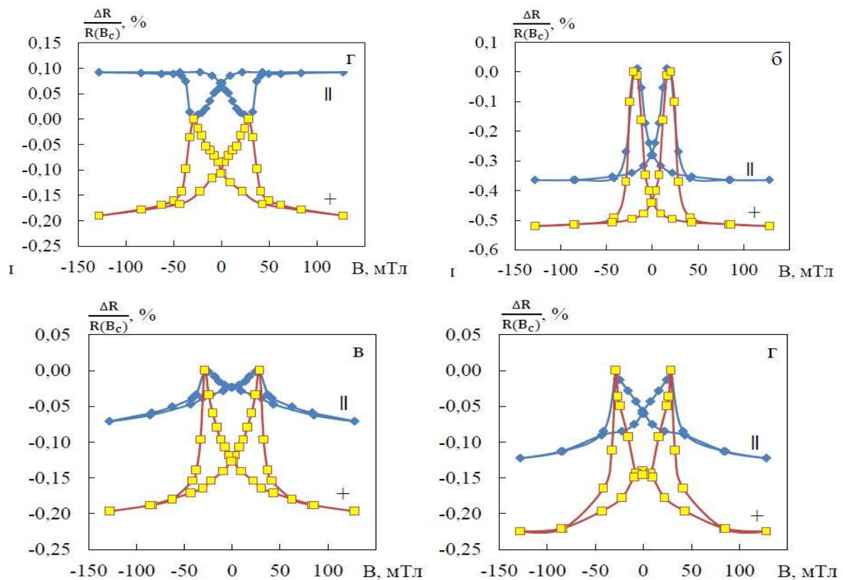
Рисунок 3.4 – Польові залежності магнітоопору для плівки сплаву (\text{Fe}_{0,8}\text{Co}_{0,2})_x\text{Cu}_{1-x}/\text{П} відпалених при температурі 550 К (а, б) і 700 К (в, г) (а – x = 0,8 , d = 40 нм; б, в, г – x = 0,5 , d_F = 40 нм). Температура вимірювання, К: 300 (а, б, в) і 100 (г)
