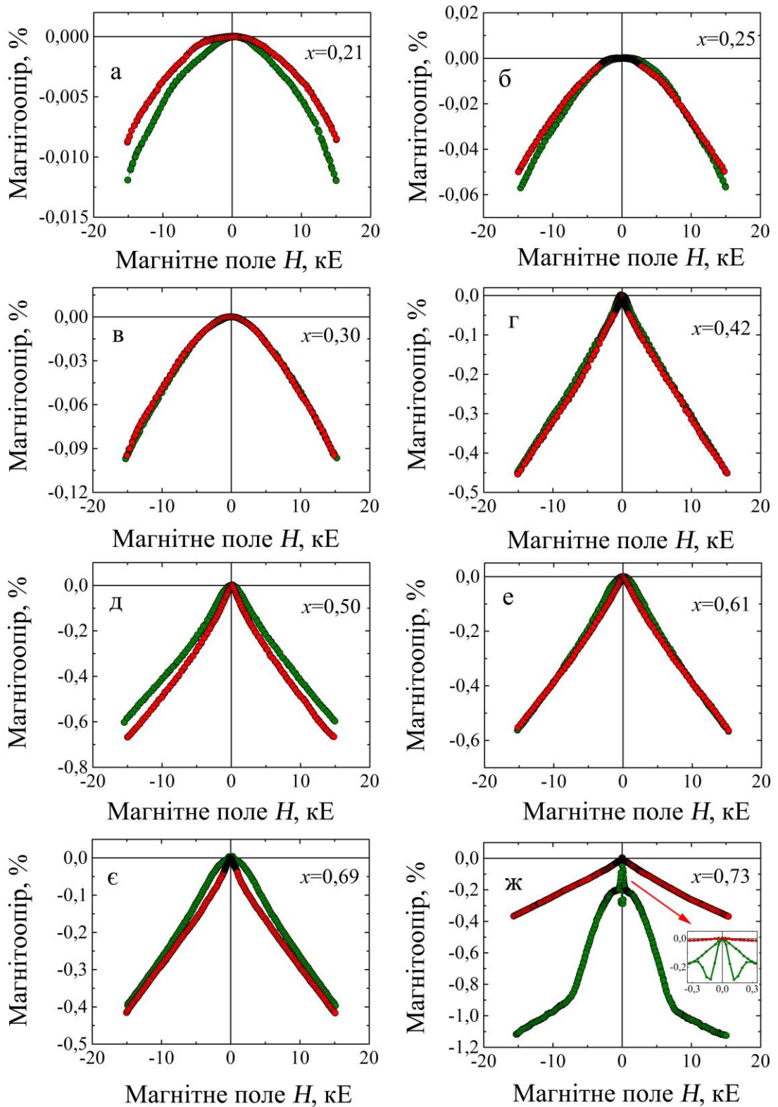
Рисунок 3.8 – Польові залежності магнітоопору невідпалених зразків плівкових сплавів на основі Рu та Сu, виміряні у перпендикулярній (●) та поздовжній (●) геометріях вимірювання при T_{\text{вимір.}} = 300 К. Товщина зразків d = 40 нм
