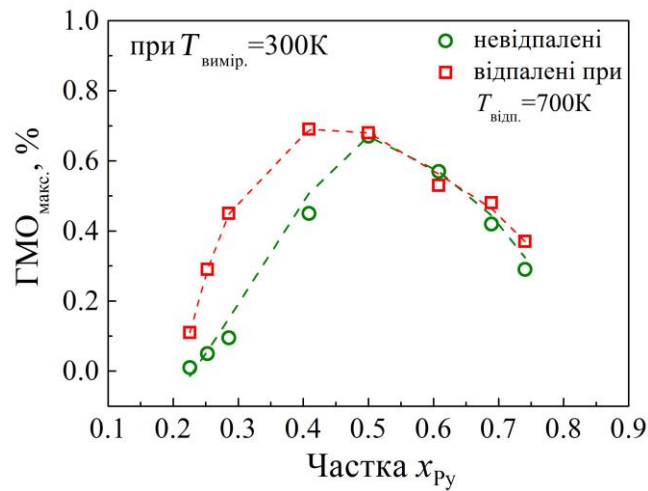
Рисунок 3.10 – Залежність величини ГМО плівкових сплавів на основі Ru і Cu товщиною d = 40 нм від їх складу у невідпаленому стані та після відпалювання при T_{\text{відп.}} = 700 К. Вимірювання ГМО здійснювали у поздовжній геометрії вимірювання у полі H_{\text{макс}} = 15 кЕ при T_{\text{вимір.}} = 300 К
