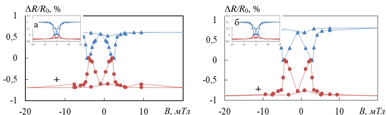
Рисунок 3.16 – Залежність поздовжнього (||) та поперечного (+) МО від індукції магнітного поля для плівок сплаву FeNiCoCu/П ( d = 60 нм; а – температура вимірювання 300 К; б – температура вимірювання 120 К)
