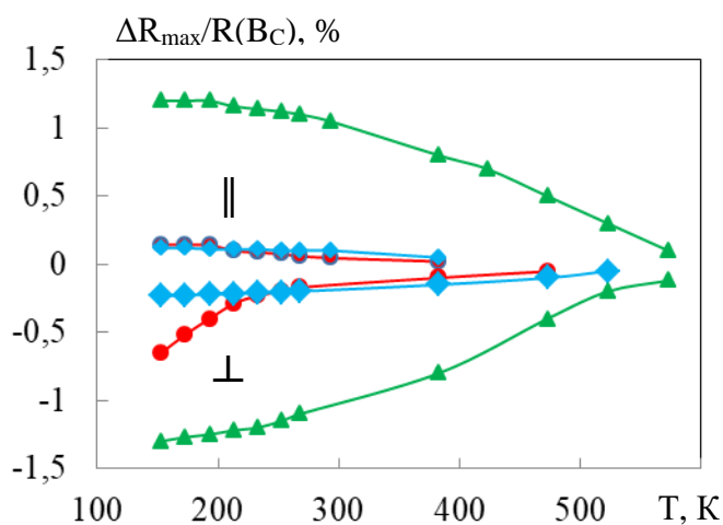
Рисунок 3.3 – Залежність поздовжнього (||) та поперечного (⊥) магнітоопору від температури вимірювання плівкових сплавів FeCo (◆), FeNi (●) та CoNi (▲)
