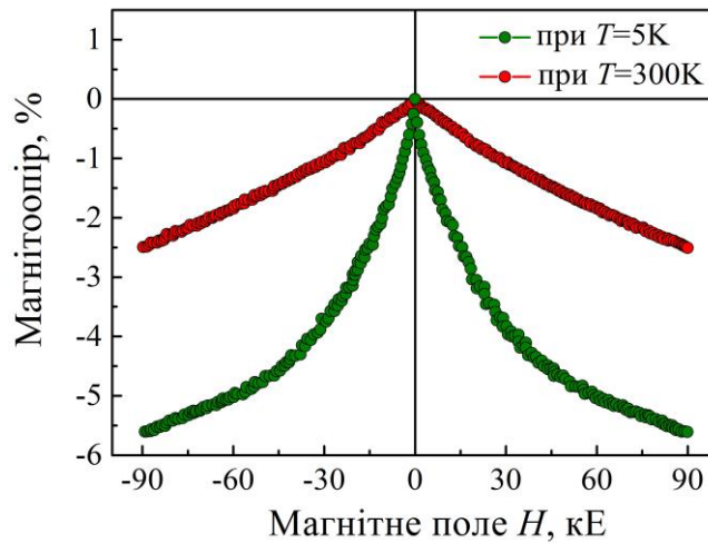
Рисунок 3.11 – Польові залежності магнітоопору невідпаленого зразка плівкового сплаву на основі пермалюю та міді з часткою пермалюю x = 0,50 . Вимірювання виконані у поздовжній геометрії при T_{\text{вимір.}} = 5 та 300 К. Товщина плівки d = 40 нм
