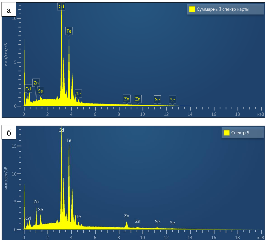
Рисунок 3.4 – Фрагменти характеристичних рентгенівських спектрів від плівок CZTS.A2 (а) та CZTS.B5 (б)
