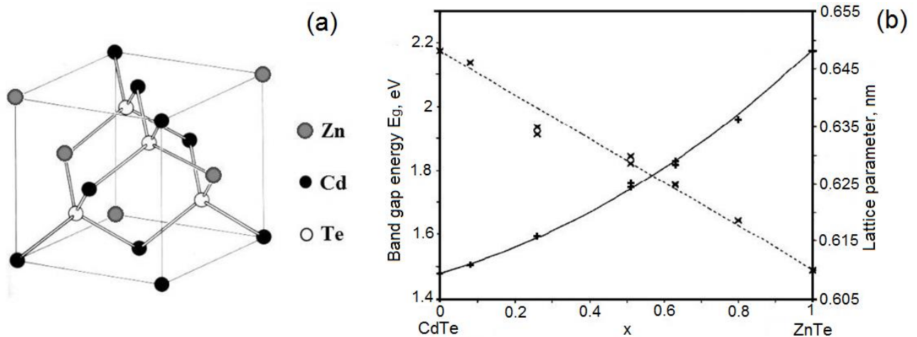
Рисунок 1.1 – Кристалічна ґратка CdTe/CZT типу сфалерит (а); та енергія забороненої зони (+) та параметр ґратки (×) за кімнатної температури як функція вмісту цинку x для твердого розчину CZT. Суцільна лінія побудована за співвідношенням 1.2; штрихована лінія – пряма апроксимуюча лінія, що з'єднує експериментальні точки [28] (б)
