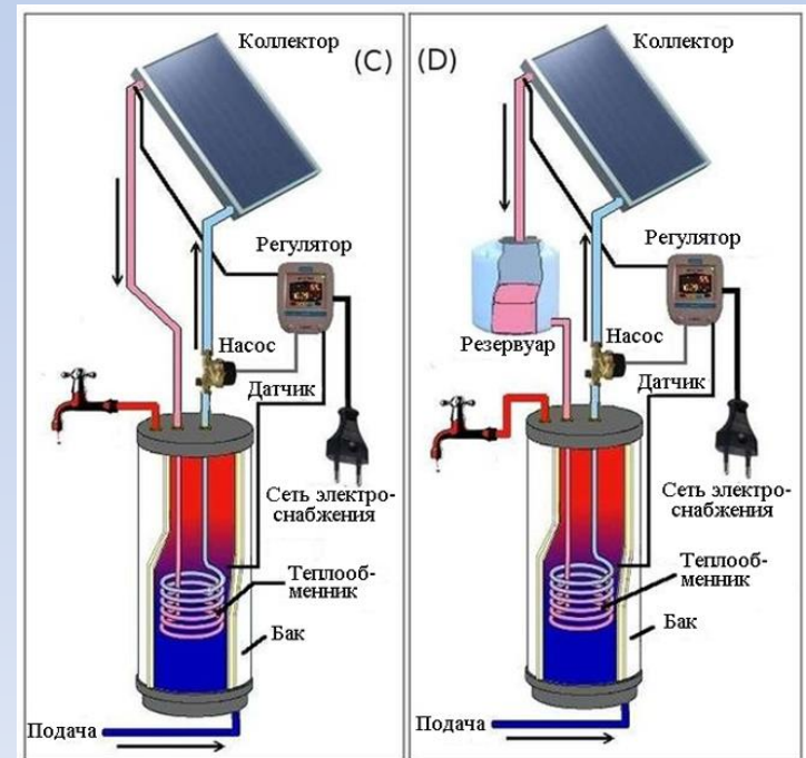
Непрямі сонячні системи
