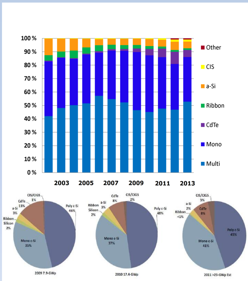
Частки ринку фотоелектричних панелей різних технологій
