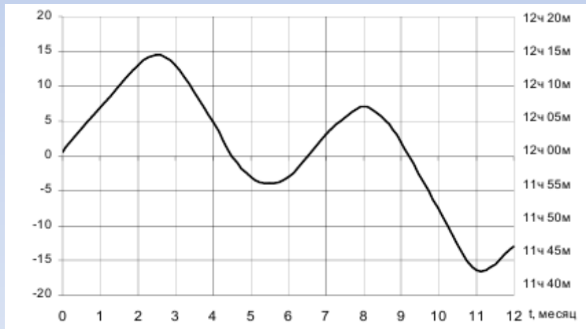
Рис. Графік рівняння часу. Крива показує середній час в істинний полудень
