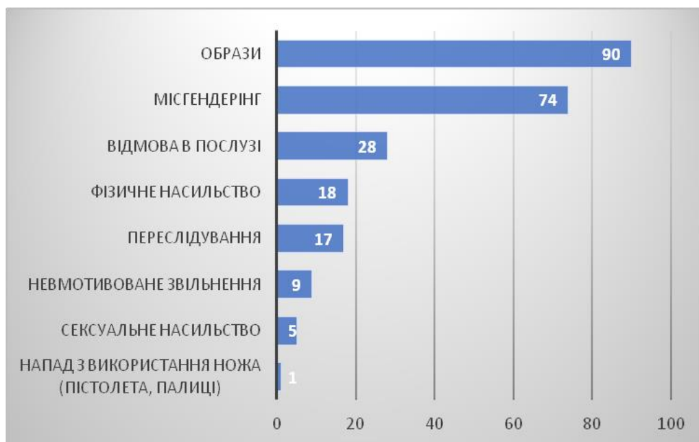
Рис. 3. Форми дискримінації/аб'юзу.
